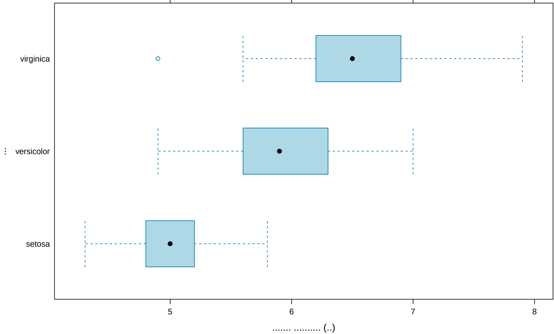
Boxplot: Sepal.Length .. .....
