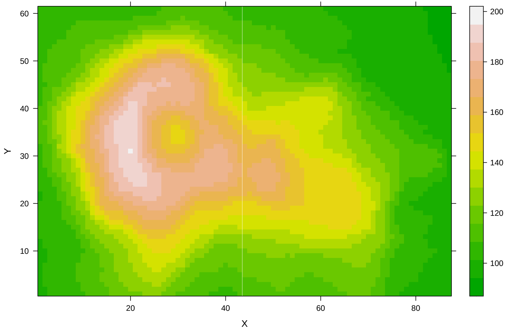
Levelplot: ..... (volcano)
