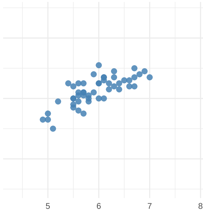
versicolor
