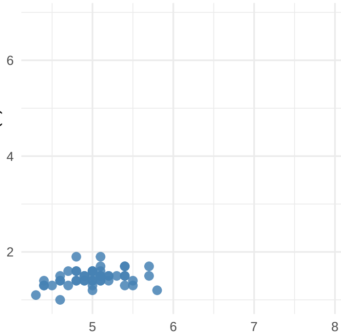
setosa
