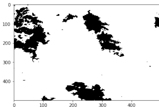
Рисунок 6.2 — Еталонна маска
