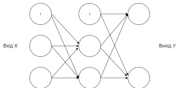
Рисунок 5. 3 - Приклад багатошарового перцептрону
