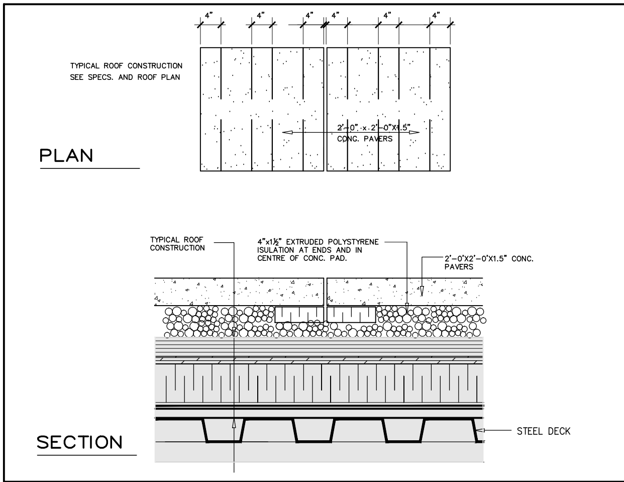
5 PAVER DETAIL SCALE: N.T.S.
