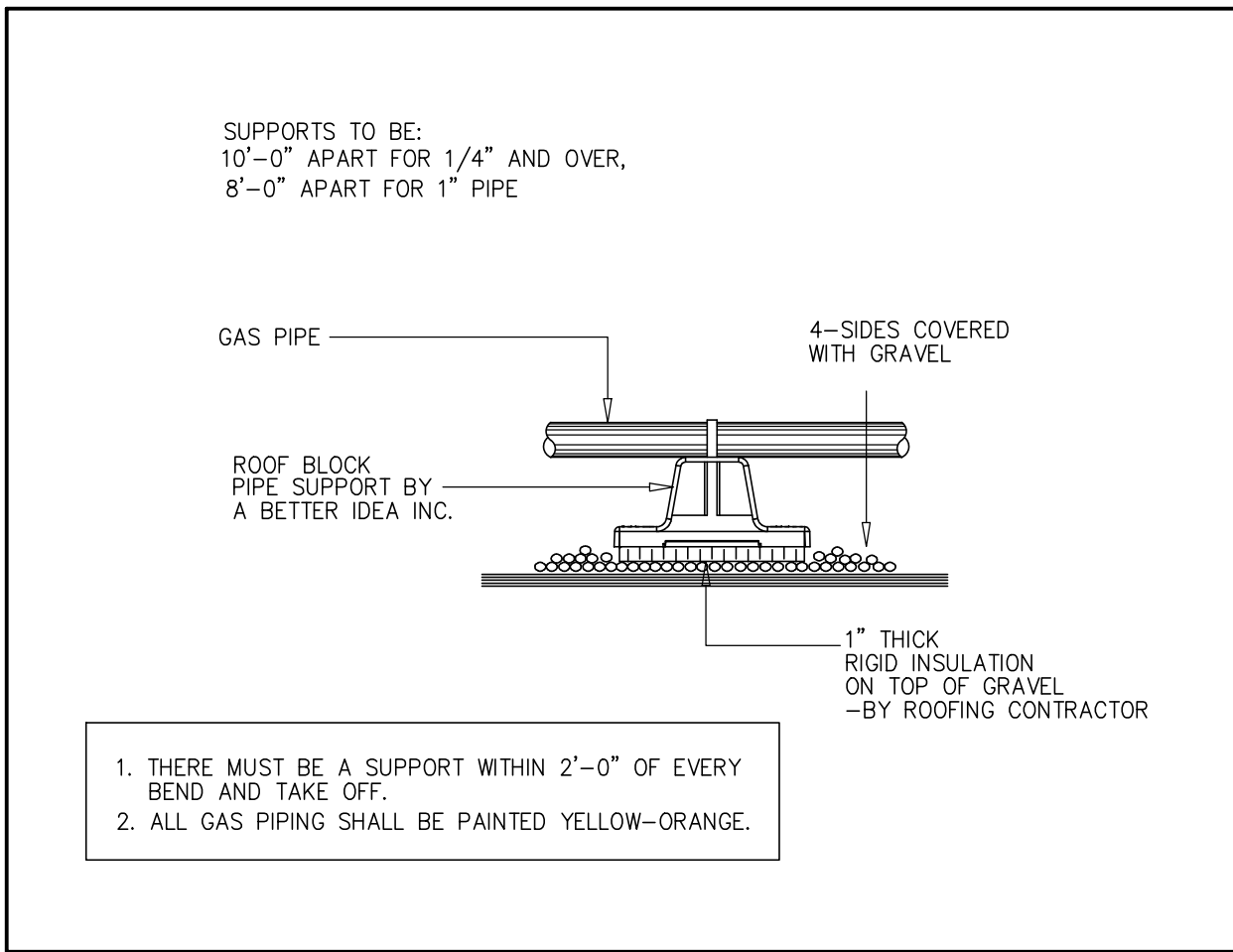
2 GAS LINE SUPPORT DETAIL SCALE: N.T.S.
