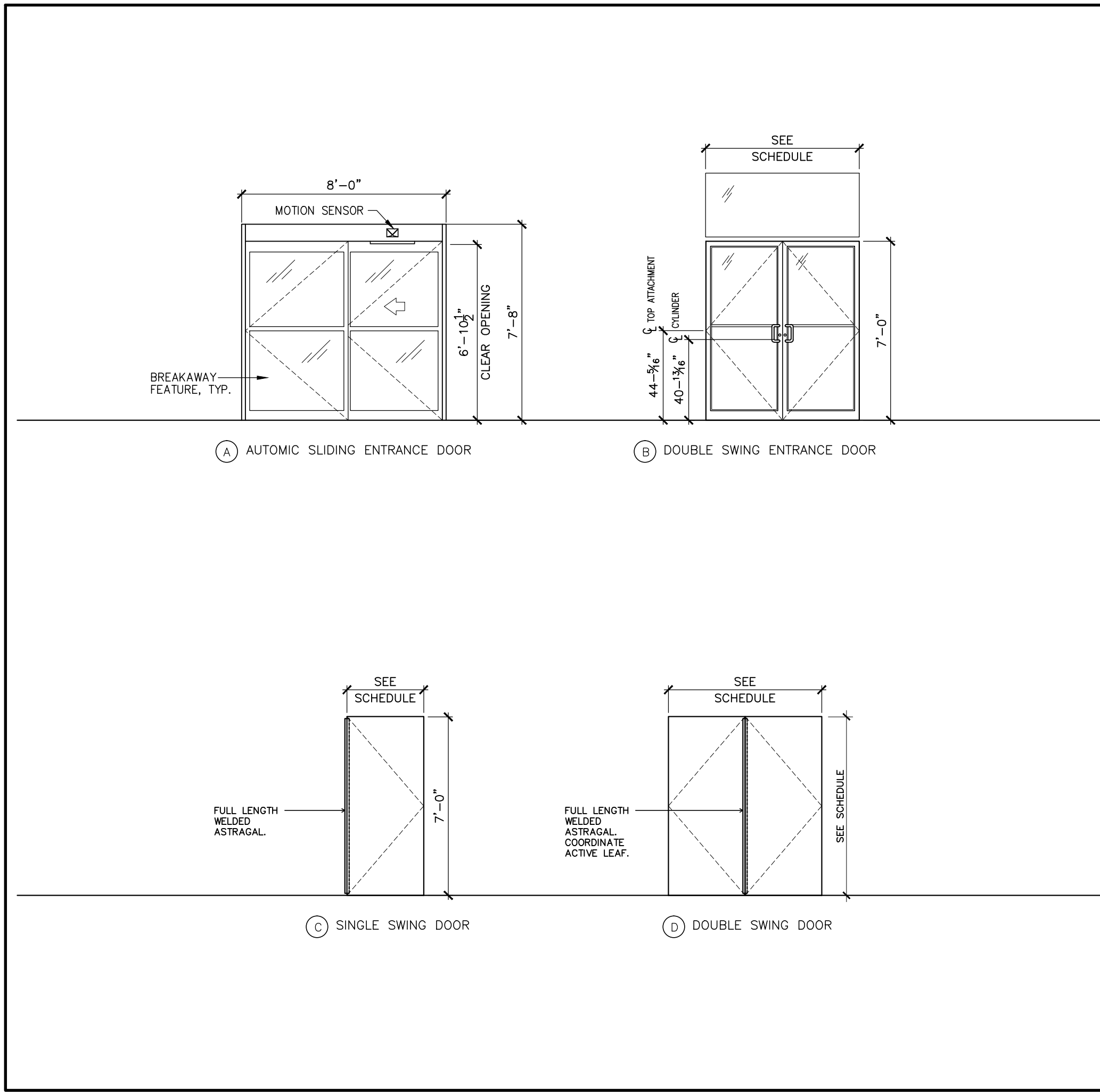
5 DOOR TYPES SCALE: N.T.S.
