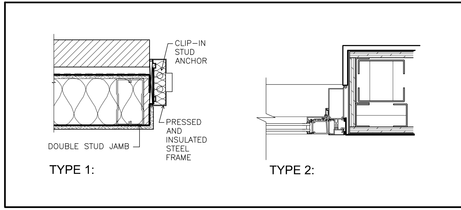
8 FRAME DETAILS/HEAD & JAMB SCALE: N.T.S.
