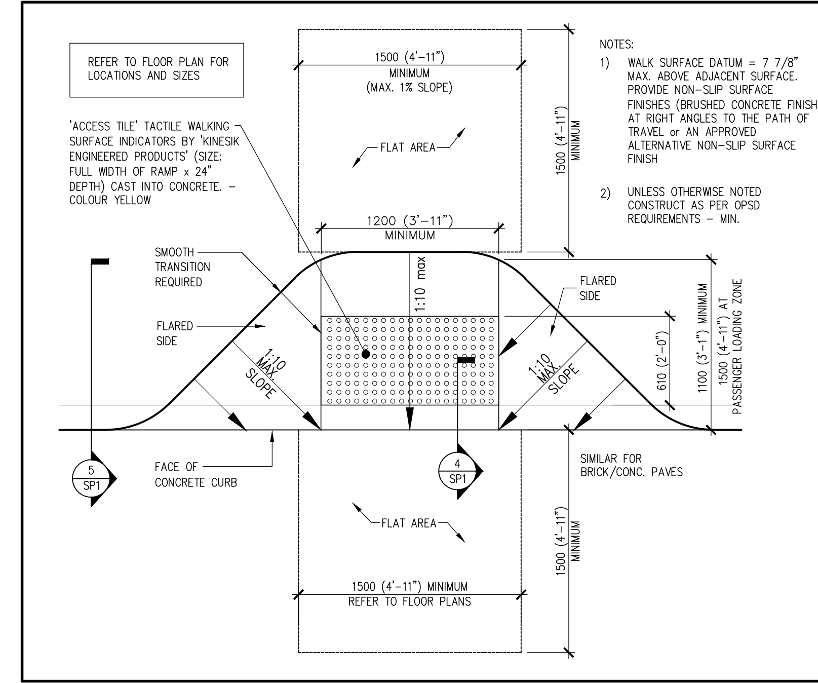
3 TYP. BARRIER-FREE RAMP PLAN SCALE: N.T.S.
