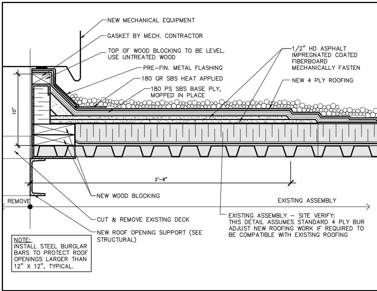
7 ROOF/R.T.U. CURB DETAIL SCALE: N.T.S.
