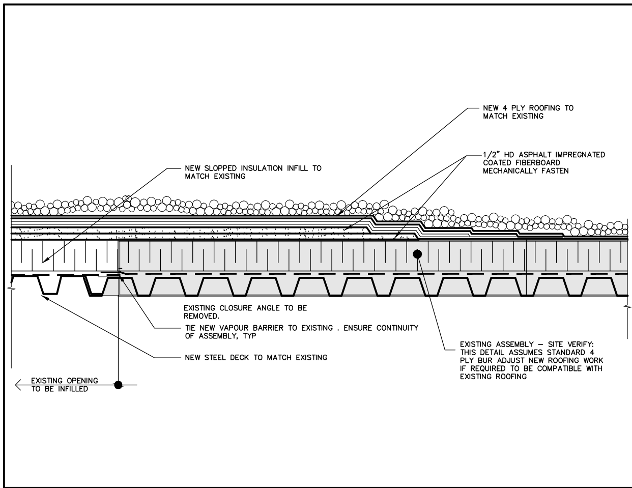
3 ROOFING DETAIL SCALE: N.T.S.
