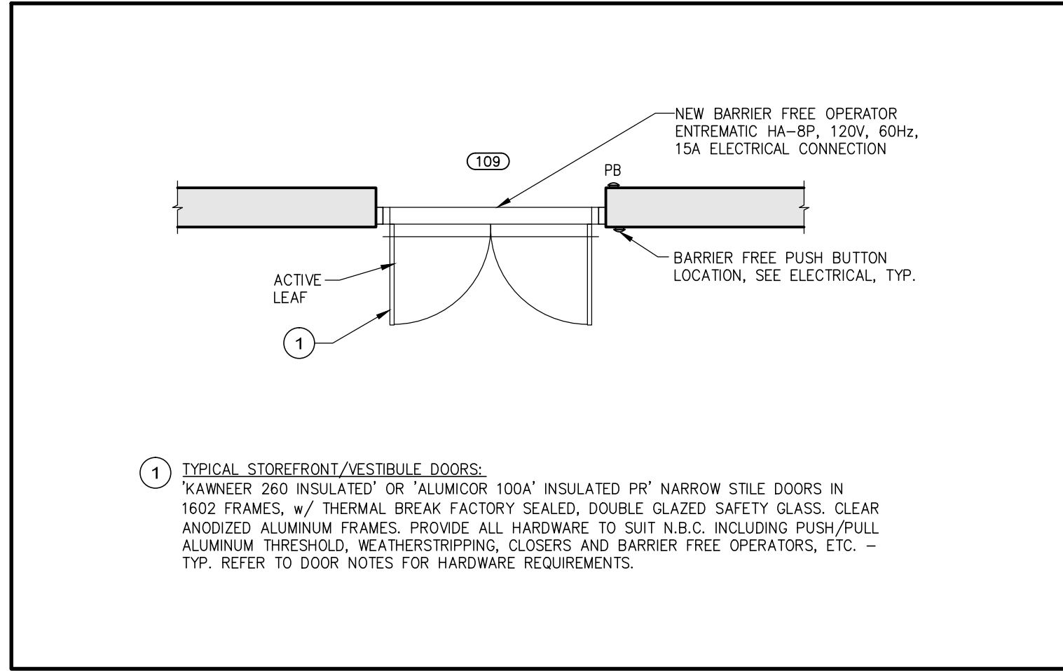
7 TYP. STOREFRONT DOOR & GLAZING SCALE: N.T.S.
