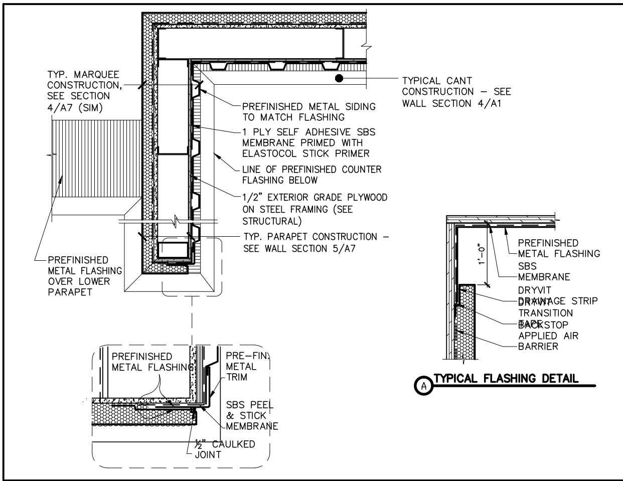
6 MARQUEE PARAPET SCALE: N.T.S.
