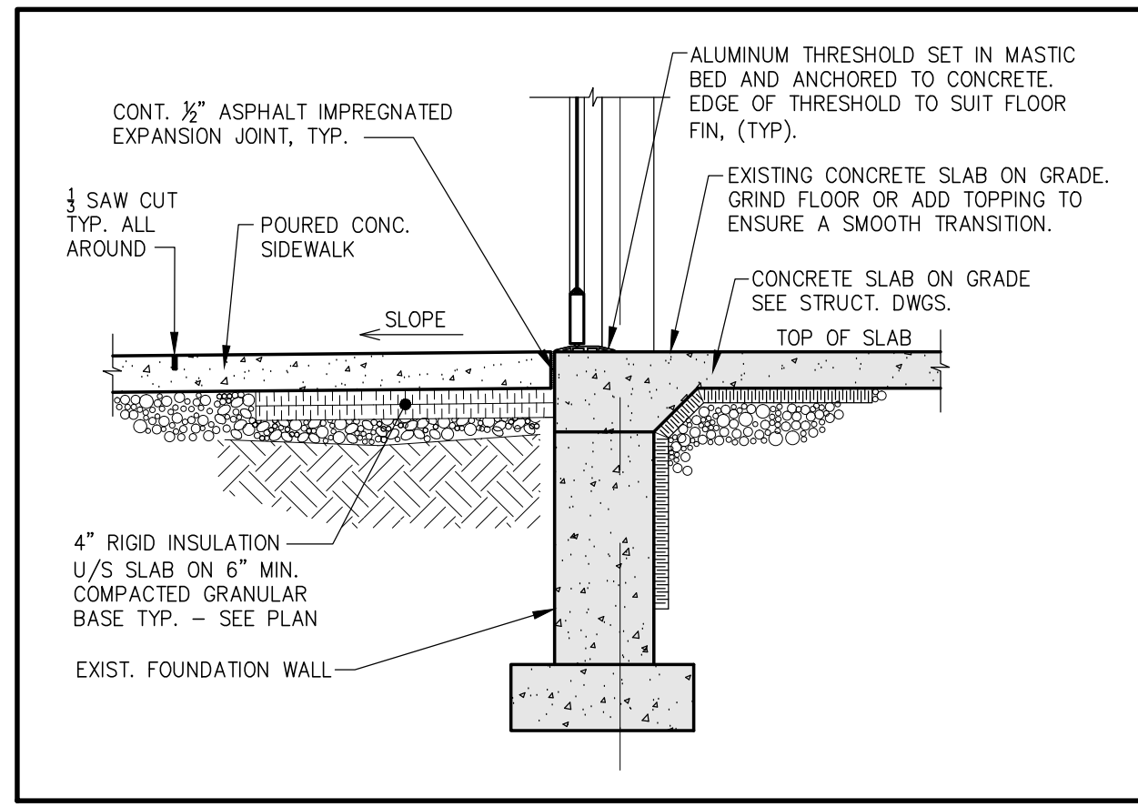
6 SECTION DETAIL @ RIGID INSULATION SCALE: N.T.S.
