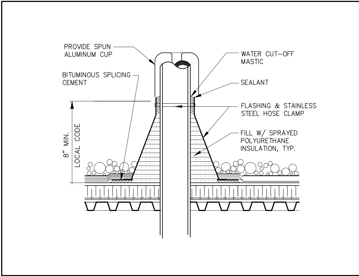
9 PIPE PENETRATION SCALE: N.T.S.
