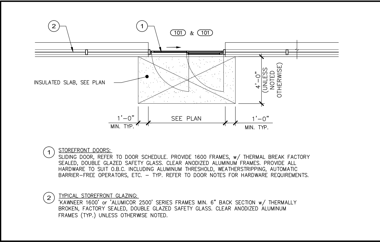
10 TYP. STOREFRONT DOOR & GLAZING SCALE: N.T.S.
