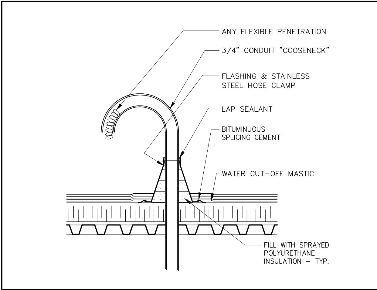
13 FLEXIBLE ROOF PENETRATION SCALE: N.T.S.
