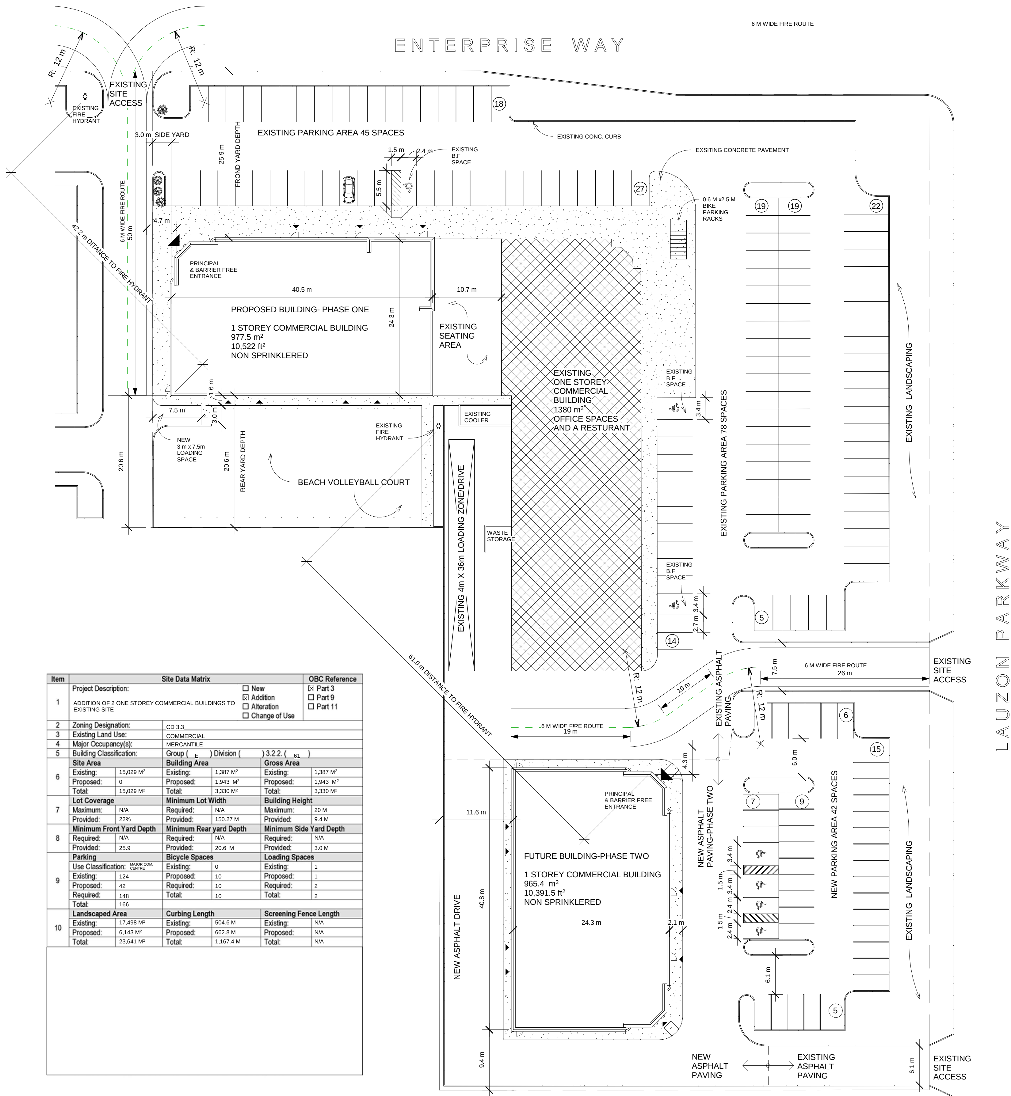
2 A001 SITE MATRIX 1 : 4
