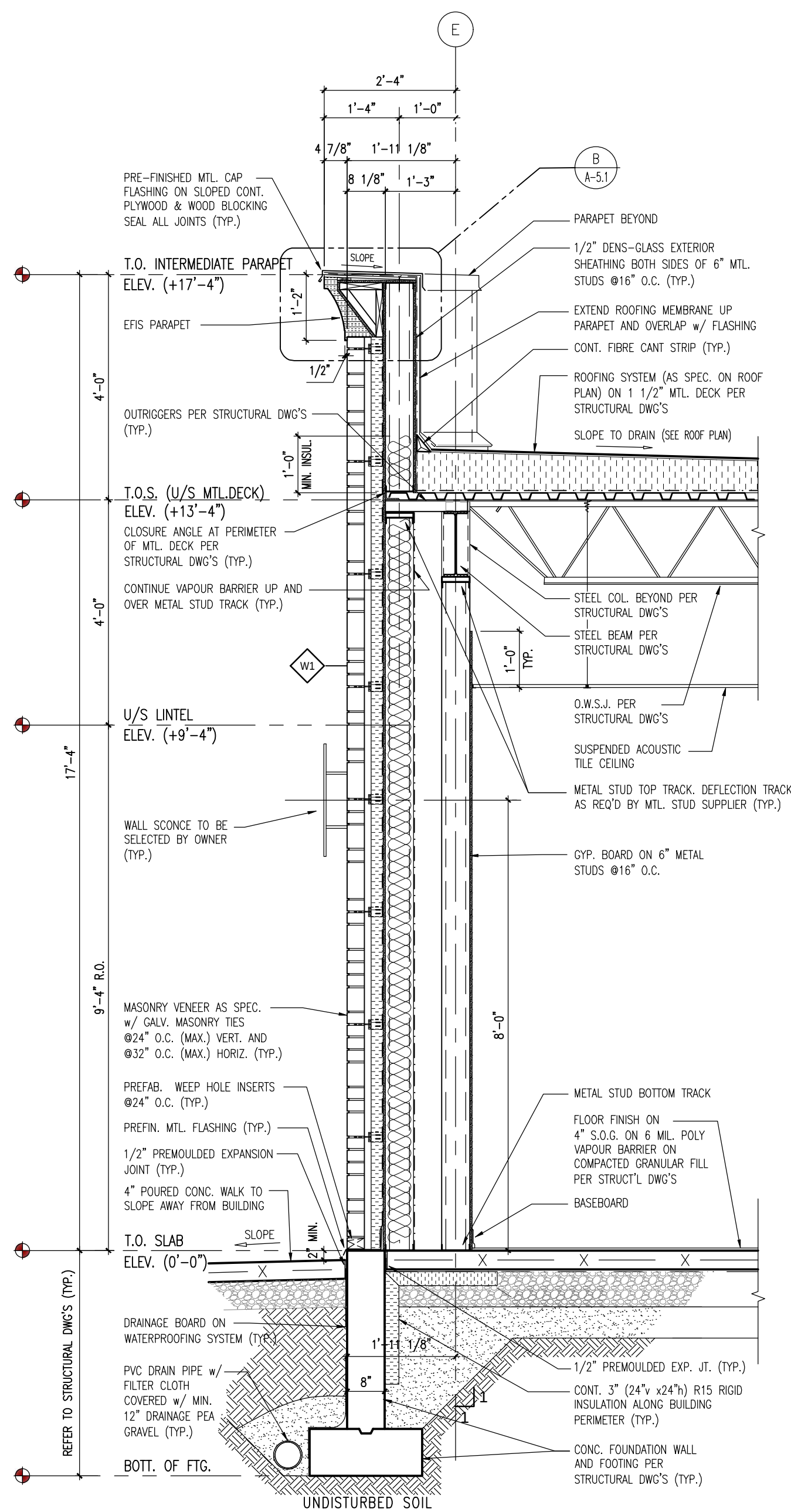
1 SECTION A-2.0, A-3.0 SCALE: 1/2" = 1'-0"
