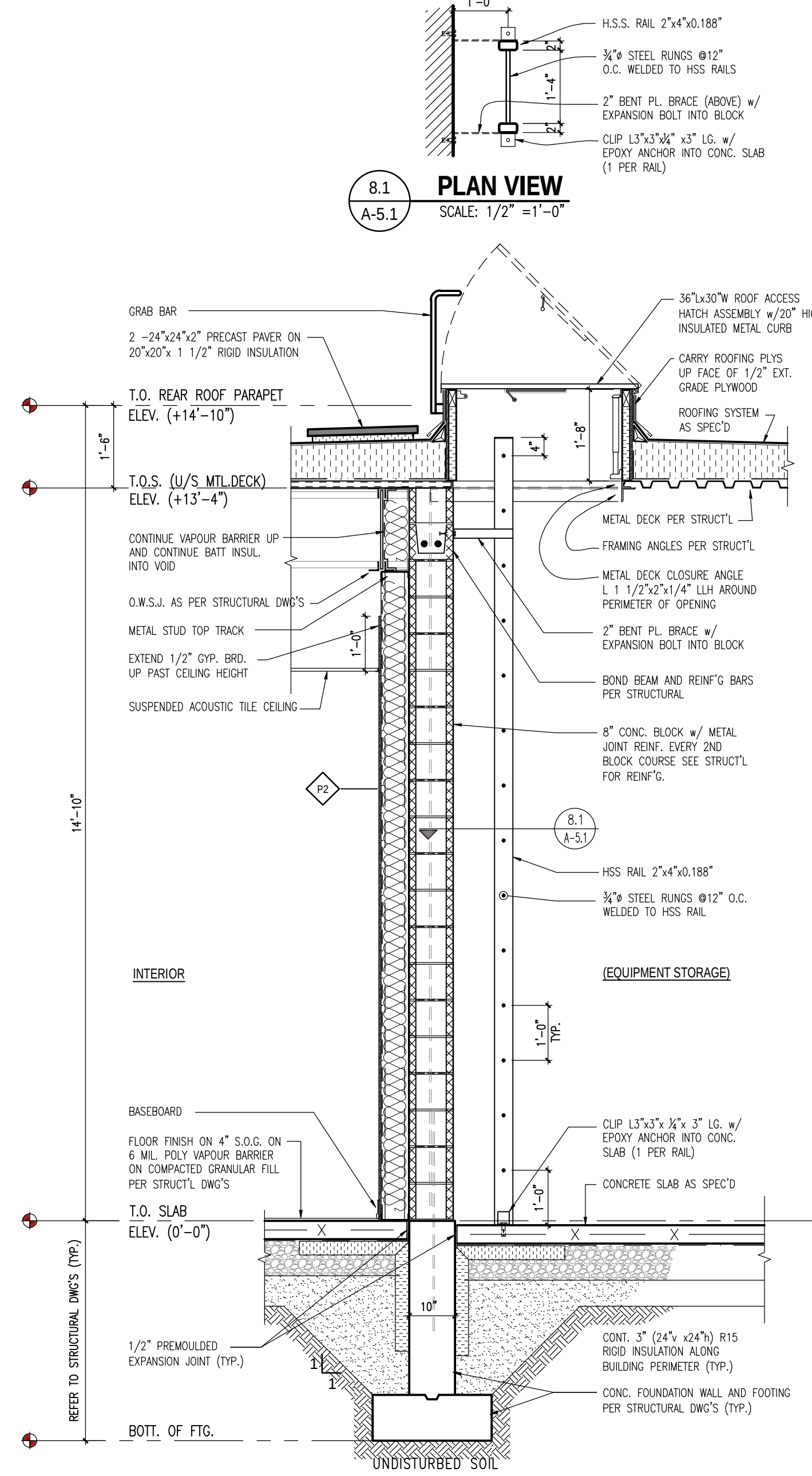
4 SECTION A-2.0, A-3.0 SCALE: 1/2" = 1'-0"
