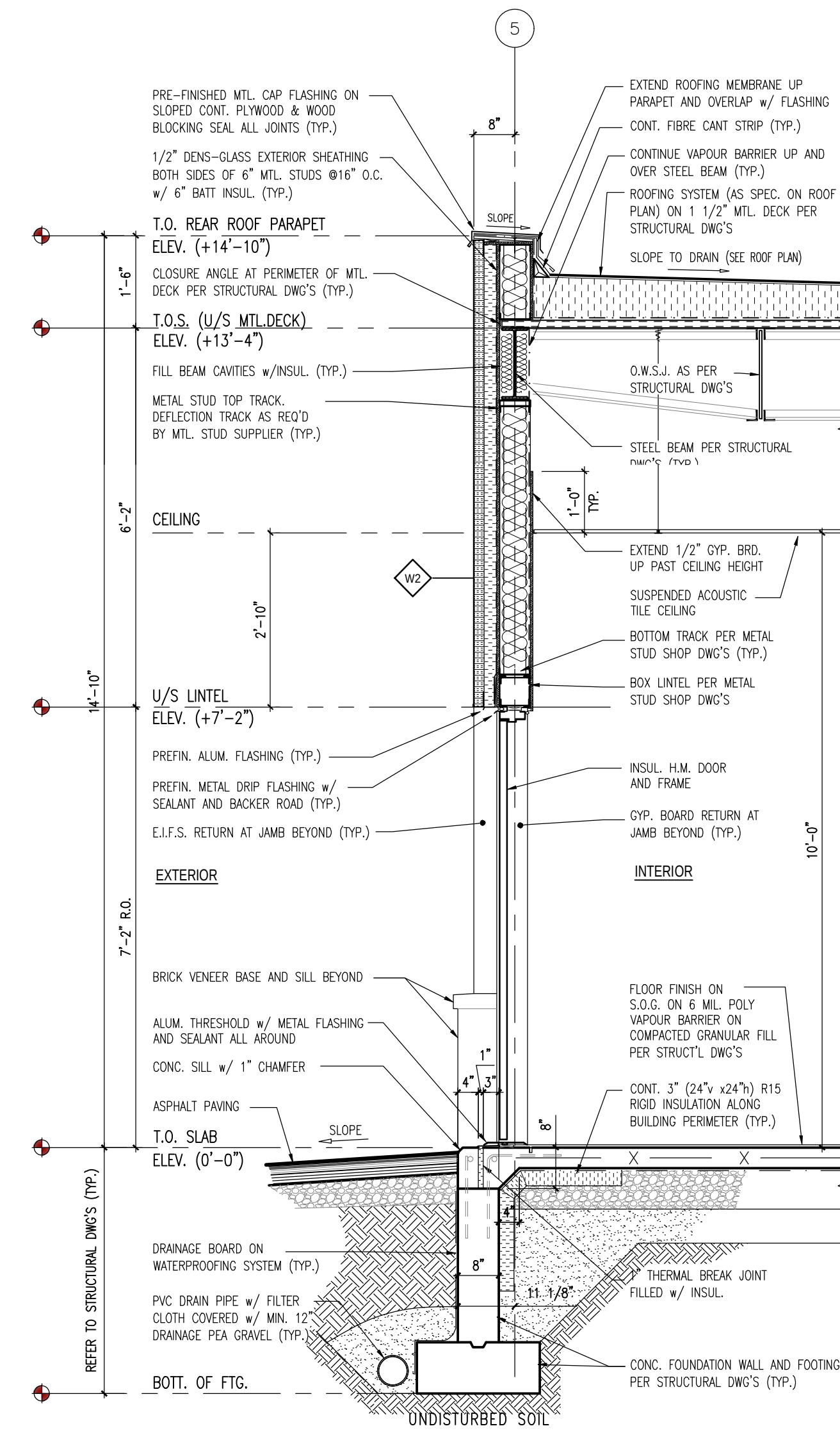
3 SECTION A-2.0, A-3.0 SCALE: 1/2" = 1'-0"
