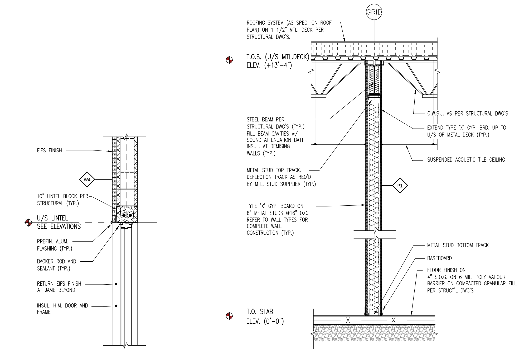
5 SECTION A-2.0 SCALE: 1/2" = 1'-0"
