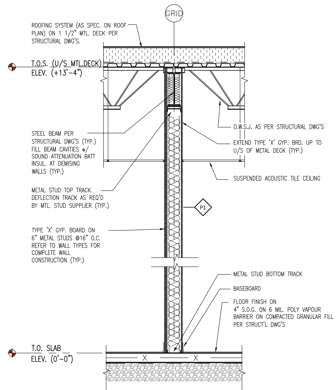
6 SECTION A-2.0, A-3.0 SCALE: 1/2" = 1'-0"
