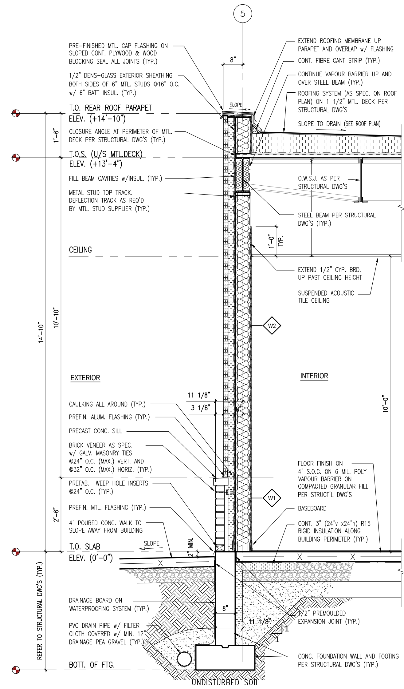
2 SECTION A-2.0, A-3.0 SCALE: 1/2" = 1'-0"
