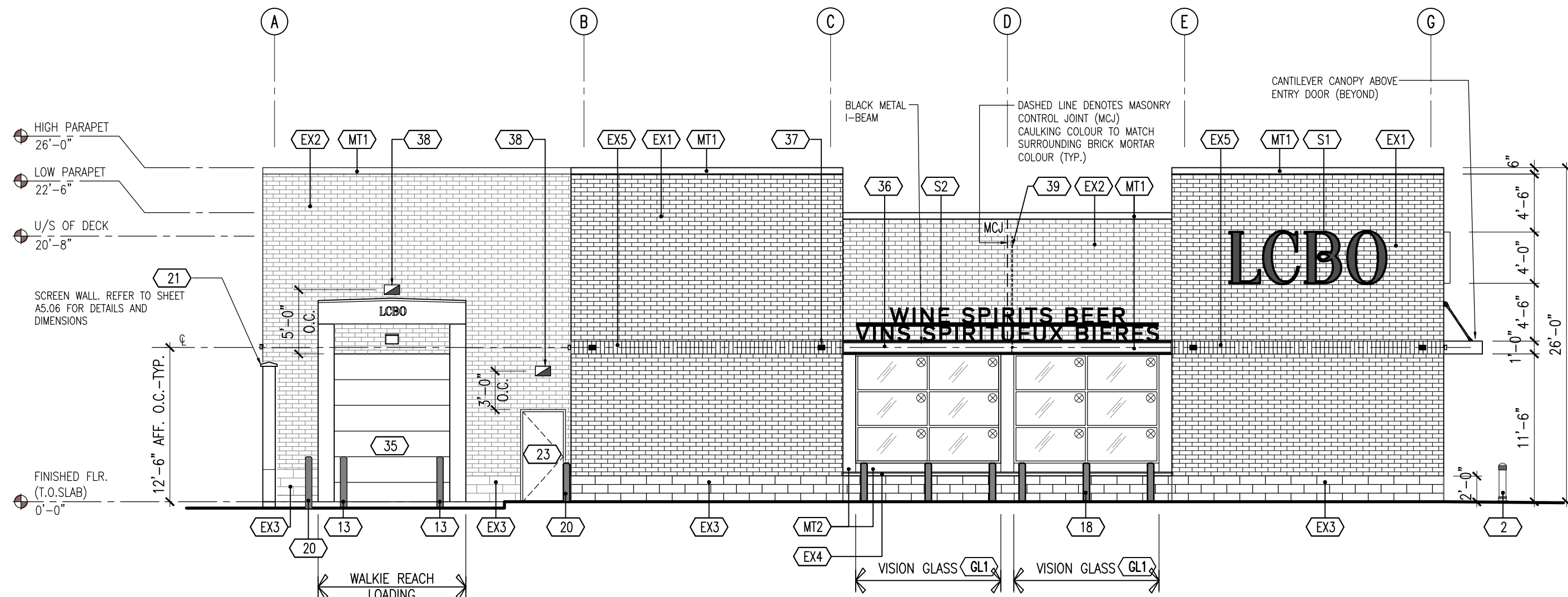
2 SOUTH ELEVATION SCALE: 1/8" = 1'-0"
