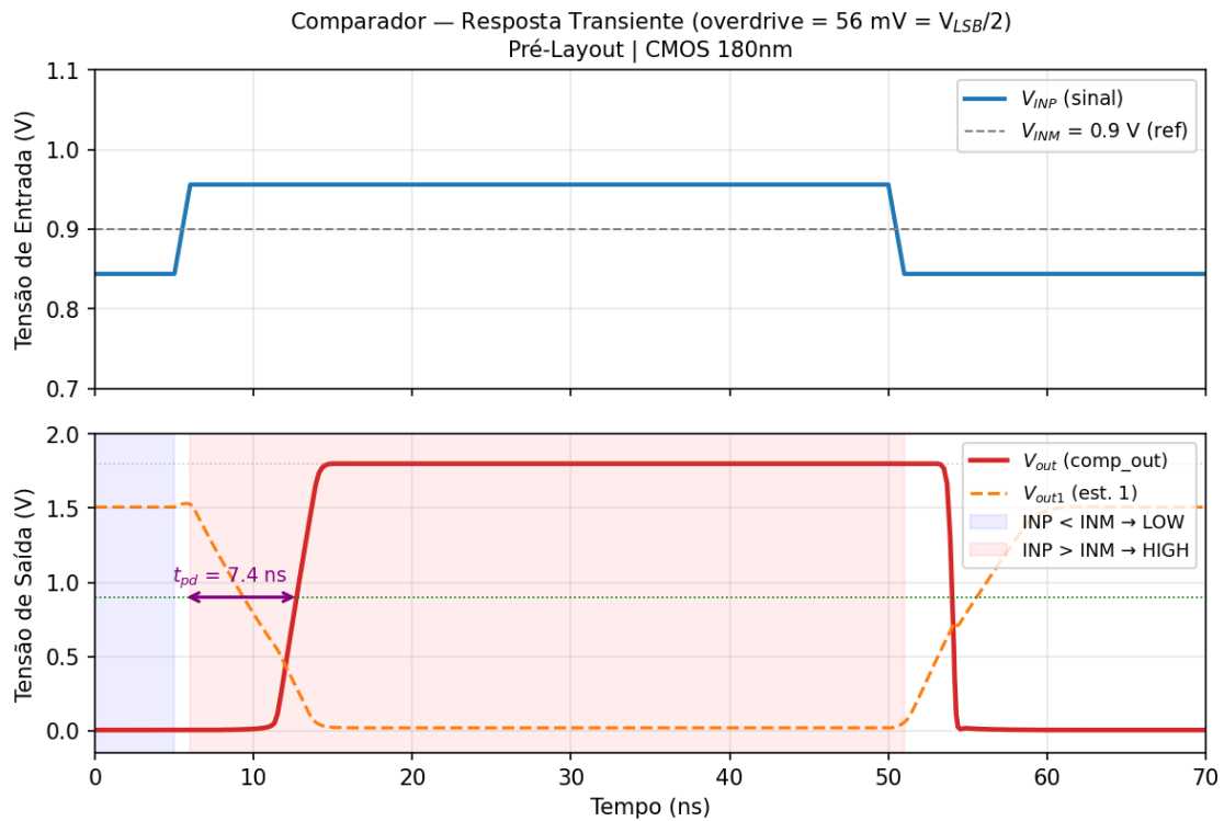
Figura 10: Resposta transiente do comparador – cenário pre-layout. Painel superior: V_{INP} com degrau de +56 mV ( = V_{LSB}/2 , overdrive mínimo) em t = 6 ns. V_{INM} = 0,900 V (referencia). Painel inferior: V_{out} (comp_out, vermelho) e V_{out1} (saida do 1º estágio, laranja tracejado). O cruzamento de V_{out} = 0,9 V ocorre em t = 13,4 ns, resultando em t_{pd} = 7,4 ns. Sem oscilacao ou metaestabilidade com overdrive mínimo de 56 mV – confirma operacao segura. A margem temporal e enorme: T_{bit}/t_{pd} = 1670/7,4 \approx 226\times .
