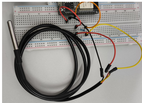
Figura 2: Sensor de temperatura DS18B20. Interface digital OneWire; GPIO 4 do ESP32. Opera em 3,3 V, faixa -55 a +125^\circ\text{C} , precisao \pm 0,5^\circ\text{C} .
