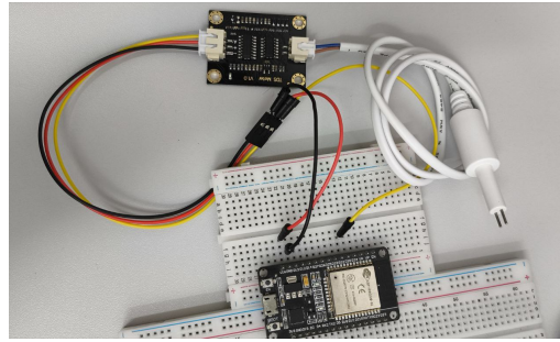
Figura 5: Modulo Gravity TDS (DFRobot). GPIO 32 do ESP32. Mede condutividade eletrica; saída analogica convertida para ppm via polinomio de 3° grau com compensacao de temperatura.
