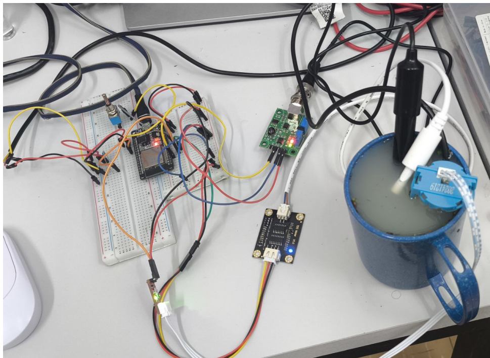
Figura 6: Montagem fisica completa do Aqua Monitor em bancada de laboratorio, mostrando o ESP32 na placa de desenvolvimento, os quatro modulos de sensores e a fiaçao de interligacao. O GPIO 27 e o pino de gatilho de coleta (ativado via MQTT ou chave manual).
