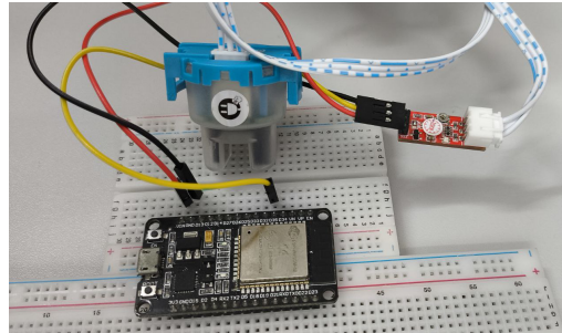
Figura 4: Sensor de turbidez SEN0189. GPIO 35 do ESP32. Mede opacidade por transmissao IR; saida 0–4,5 V inversamente proporcional a turbidez em NTU.
