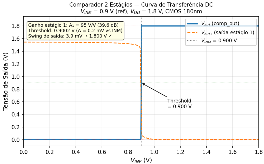
Figura 9: Curva de transferencia DC do comparador. V_{INP} varre de 0 a 1,8 V com V_{INM} = 0,9\text{ V} fixo. A tensão de comutacao medida pelo Ngspice e V_{th} = 900,2\text{ mV} (desvio de apenas 0,2\text{ mV} frente a V_{INM} , atribuível ao descasamento dos modelos Level-1). A excursao de saída V_{out} vai de 3,9\text{ mV} (LOW, M6 em sub-tensão) a 1,800\text{ V} (HIGH, M7 em triodo) – saída de trilho a trilho. O ganho de malha aberta medido na região de transicao e \approx 95\text{ V/V} = 39,6\text{ dB} , confirmando o calculo teorico.
