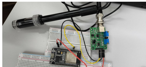
Figura 3: Modulo PH4502C com eletrodo de vidro. GPIO 34 do ESP32; saida analogica 0–3 V. Requer calibracao em tampoes de pH 4 e pH 7.
