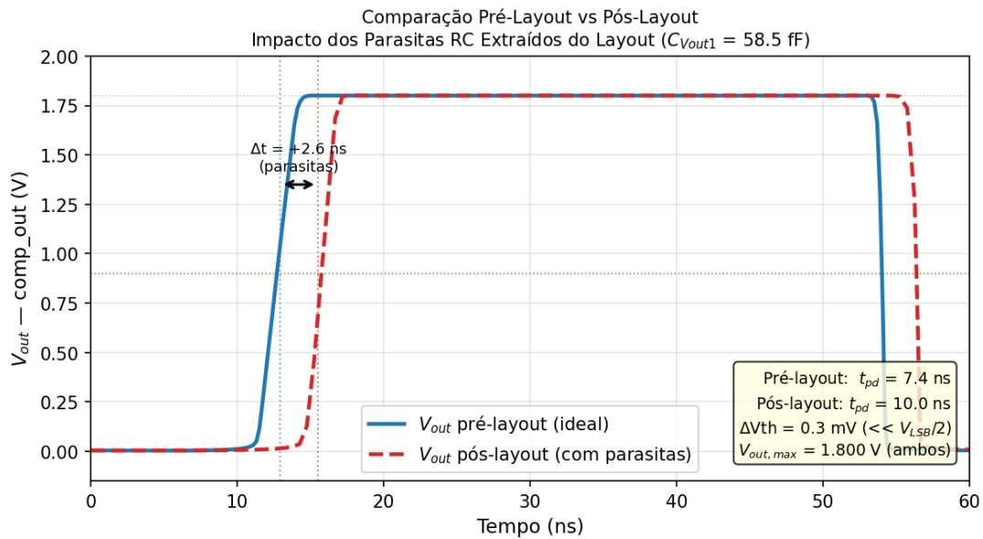
Figura 11: Comparacao pre-layout vs. pos-layout. A inclusao dos parasitas RC extraídos do GDS causa uma degradacao do tempo de propagacao de 7,4ns para 10,0ns ( \Delta = +2,6 \text{ ns} , correspondente a apenas 0,6% do periodo do SAR de 1,67 \mu\text{s} ). O nivel de saida maximo de 1,800 V e preservado em ambas as versoes. A variacao do limiar de comutacao e \Delta V_{th} = 0,3 \text{ mV} < V_{LSB}/375 – os parasitas nao alteram a decisao de nenhum bit. O resultado confirma a robustez do projeto para tape-out.
