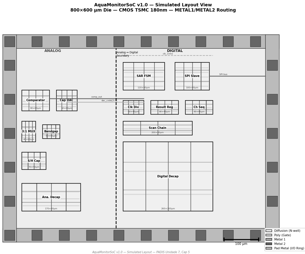
Figura 12: Vista de layout simulada – camadas de difusão, poli, Metal1 e Metal2. Canais de roteamento entre blocos e escala de 100 \mu\text{m} .
