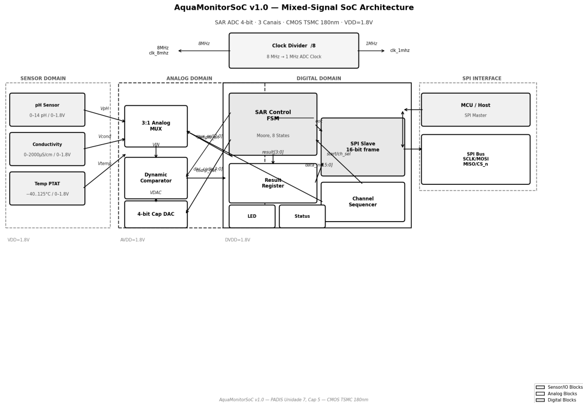
Figura 9: Visão de sistema do AquaMonitorSoC v1.0 – interconexão dos blocos conforme implementado no top-level.
