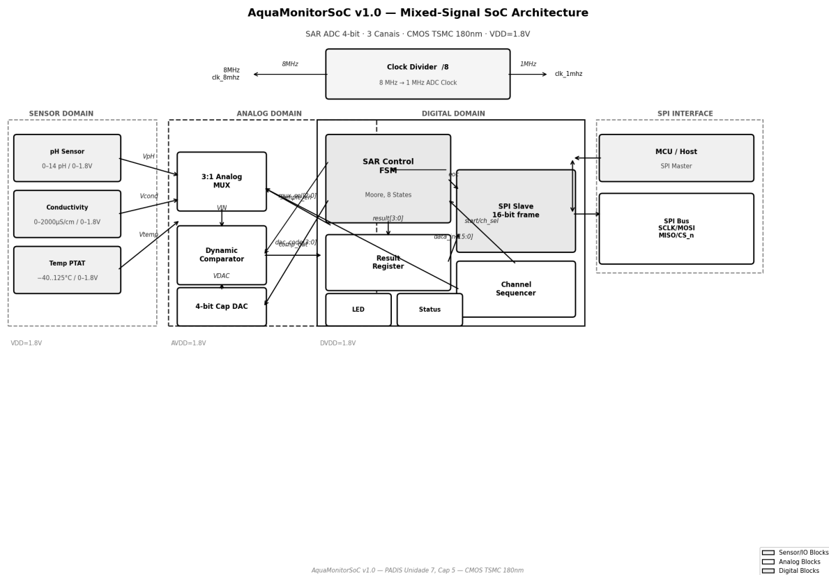
Figura 2: Arquitetura completa do AquaMonitorSoC v1.0. Blocos sensoriais (esquerda), domínio analógico interno (centro) e domínio digital (direita).
