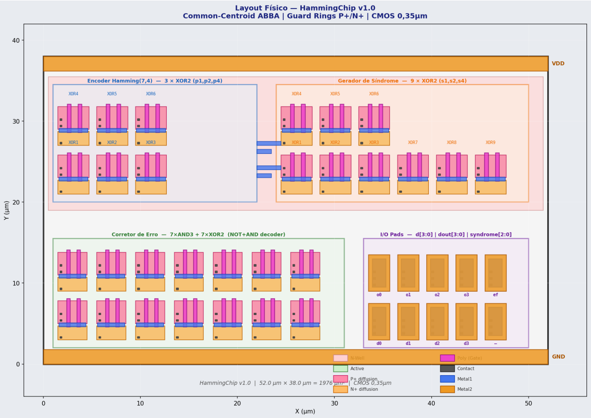
Figura 10: Layout físico de die do HammingChip v1.0 (52 μm × 38 μm, CMOS 0,35 μm). Blocos: Encoder (azul), Síndrome (laranja), Corretor (verde), I/O Pads (roxo). Metal-2 nos trilhos VDD/GND.
