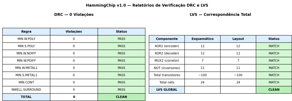
Figura 13: Relatório de verificação DRC e LVS: zero violações detectadas.
