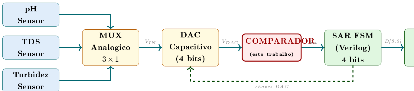
Figura 6: Cadeia de sinais completa do SAR ADC no sistema AquaMonitor. O comparador diferencial (destacado em vermelho) e o bloco analogico central projetado neste trabalho. O DAC capacitivo (5 capacitores MIM, C_{tot} = 1600 fF) e a FSM SAR (Verilog) completam o conversor de 4 bits.
