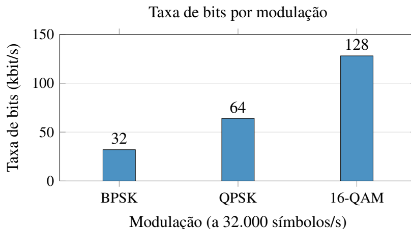
Figura 13: Taxa de bits para taxa de símbolos fixa em 32.000 símbolos/s
