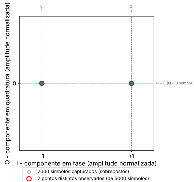
Figura 3: Constelação BPSK observada no plano I/Q
