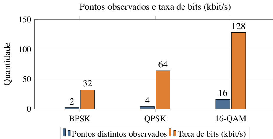
Figura 11: Comparação entre as três modulações a 32.000 símbolos/s
