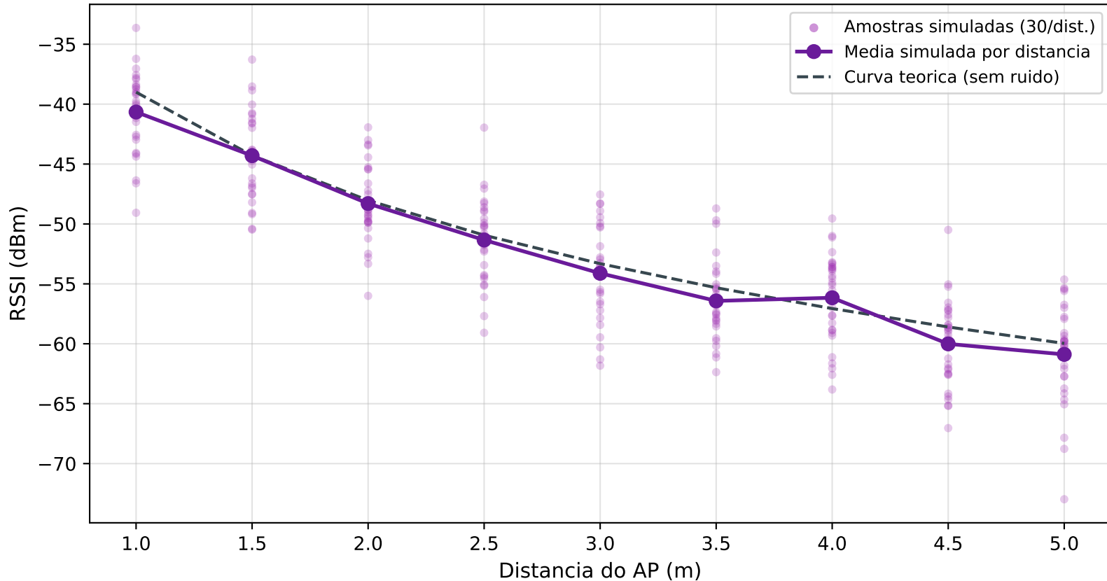
Modelo Log-Distance - RSSI simulado em funcao da distancia Pt=20 dBm, n=3.0, sigma=4 dB
