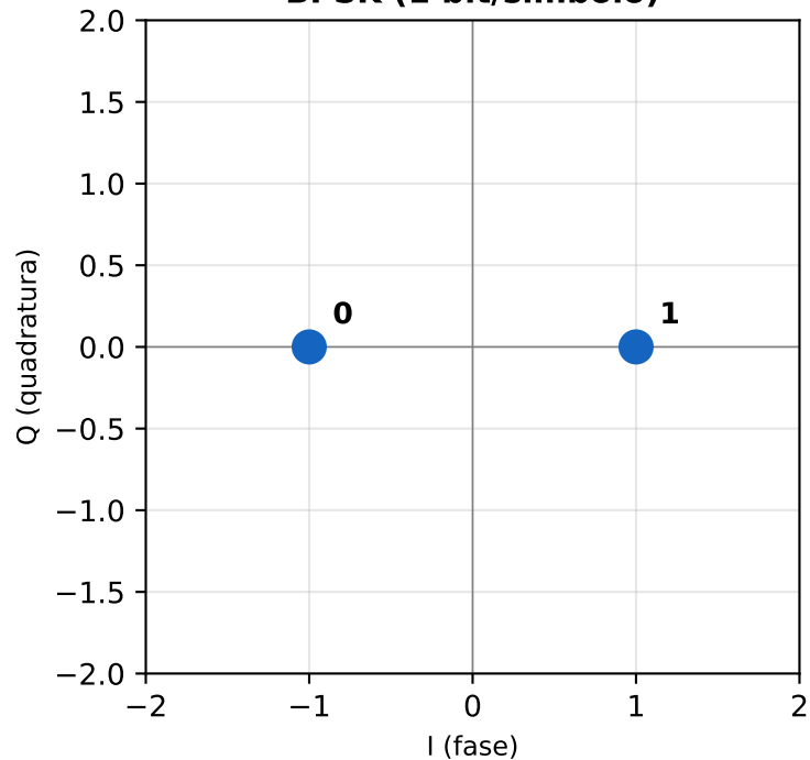
BPSK (1 bit/simbolo)
