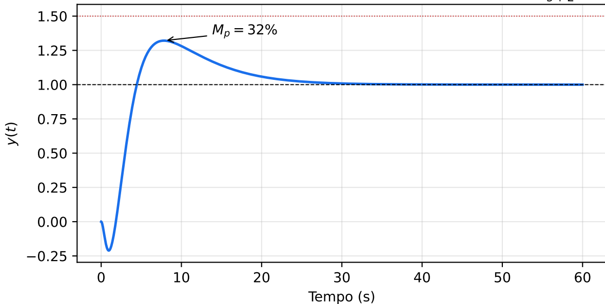
Resposta ao degrau — malha fechada com C(s) = -2 \frac{s+0,1}{s+2}
