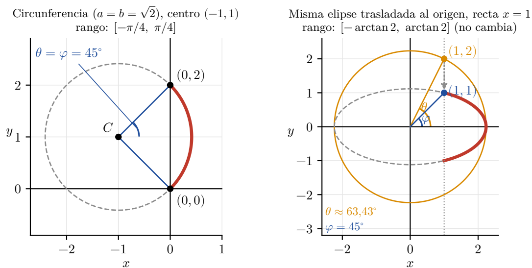
Figura 4: Izquierda: circunferencia de centro (-1, 1) que pasa por (0, 0) y (0, 2) ; el parámetro coincide con el ángulo polar ( 45^\circ ). Derecha: la elipse del ejercicio trasladada al origen; el rango sigue siendo [-\arctan 2, \arctan 2] .
