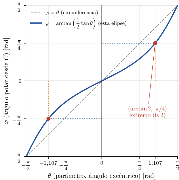
Figura 3: Ángulo polar \varphi en función del parámetro \theta para b/a = 1/2 , comparado con la circunferencia ( \varphi = \theta ). Ambos coinciden solo en 0 y \pm\pi/2 .
