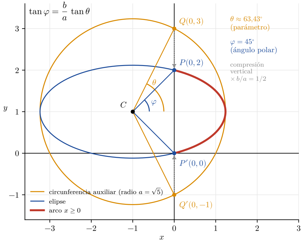
Figura 2: Circunferencia auxiliar de radio a = \sqrt{5} . La compresión vertical de factor b/a = 1/2 lleva Q a P y Q' a P' : el parámetro mide \theta \approx 63,43^\circ en la circunferencia, mientras que el ángulo polar del punto de la elipse es \varphi = 45^\circ .
