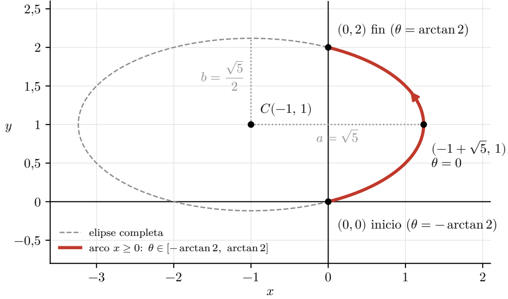
Figura 1: Elipse \frac{(x+1)^2}{5} + \frac{(y-1)^2}{5/4} = 1 y arco x \geq 0 (en rojo), recorrido en sentido antihorario para \theta \in [-\arctan 2, \arctan 2] .
