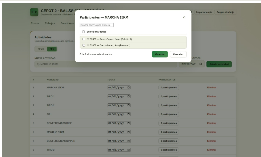
Fig. 13 — Actividades: buscador de participantes de una actividad, con selección individual o de todos.
