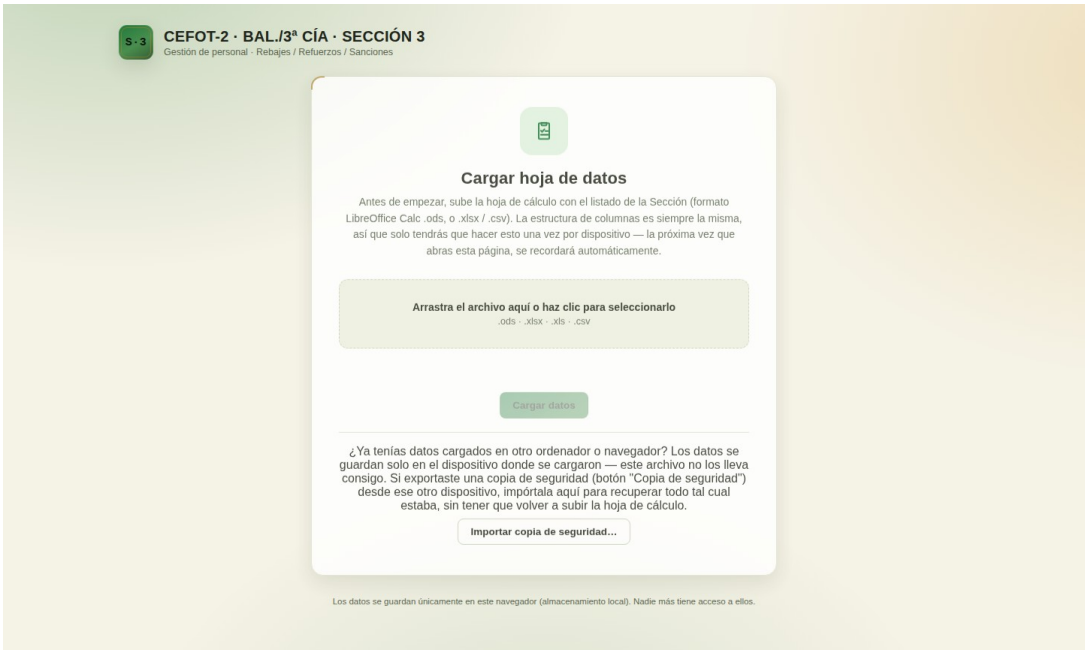
Fig. 1 — Pantalla inicial: recuadro de carga del listado y acceso a la importación de una copia de seguridad.
