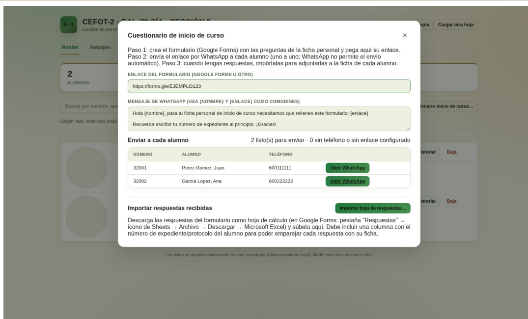
Fig. 5 — Cuestionario de inicio de curso: enlace del formulario, envío por WhatsApp alumno a alumno e importación de respuestas.
