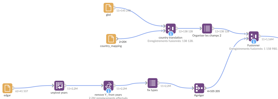
FIGURE 23 – Pipeline de préparation des données dans Omniscope
