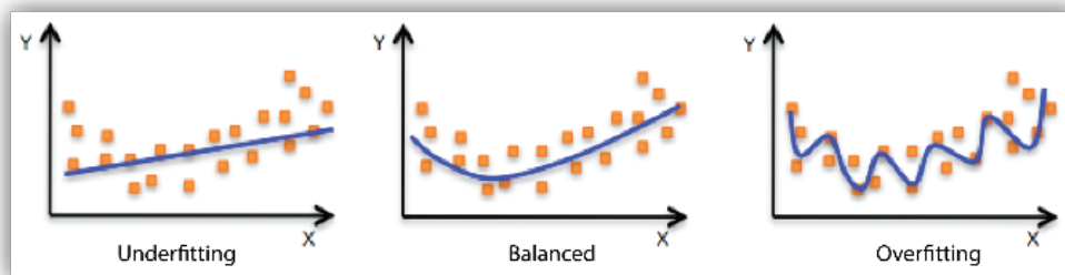
Fig. 20. – Overfitting et Underfitting : illustration des deux extrêmes
