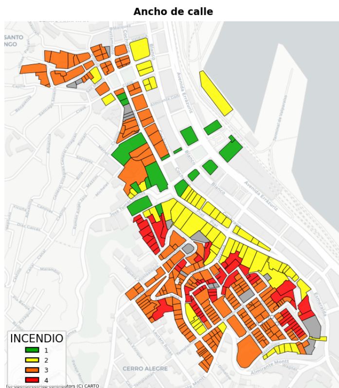
ANCHO DE CALLE Nº; % DE EDIFICIOS
