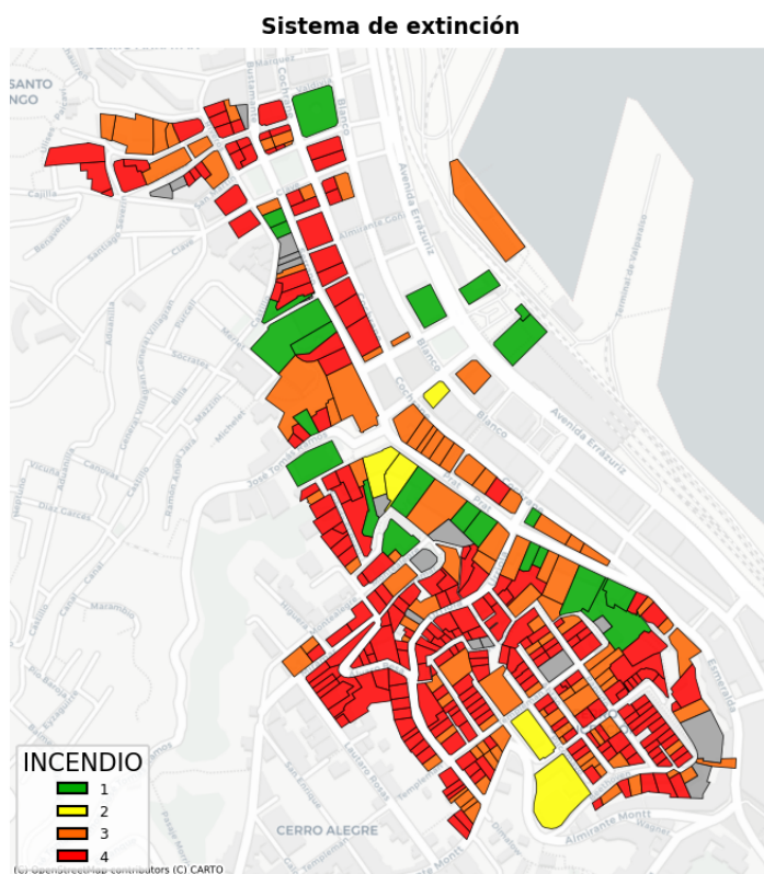
SISTEMA DE EXTINCIÓN Nº; % DE EDIFICIOS
