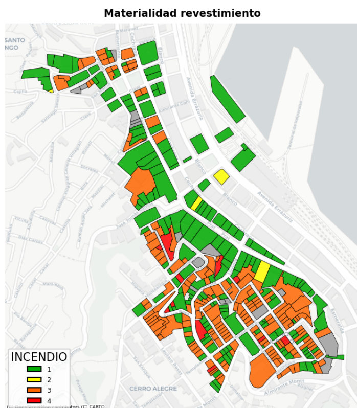
MATERIALIDAD REVESTIMIENTO Nº; % DE EDIFICIOS
