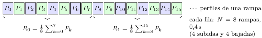
Figura 9.7: Formación de las filas del radargrama a partir de los perfiles de cada rampa. En azul las subidas, en verde las bajadas invertidas; cada fila mezcla las dos.
