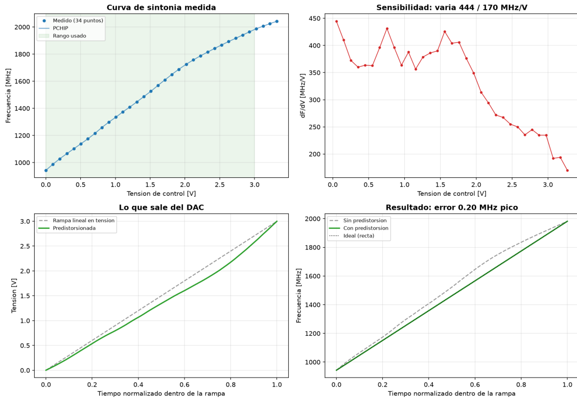
Figura 5.2: Linealización del barrido del VCO mediante predistorsión (script VCO/analisis_vco.py ). Arriba: curva de sintonía medida con ajuste PCHIP (izq.) y sensibilidad dF/dV punto a punto sin suavizar (der.). Abajo: rampa de tensión del DAC con y sin predistorsión (izq.) y frecuencia resultante en función del tiempo normalizado, comparada con la recta ideal (der.).
