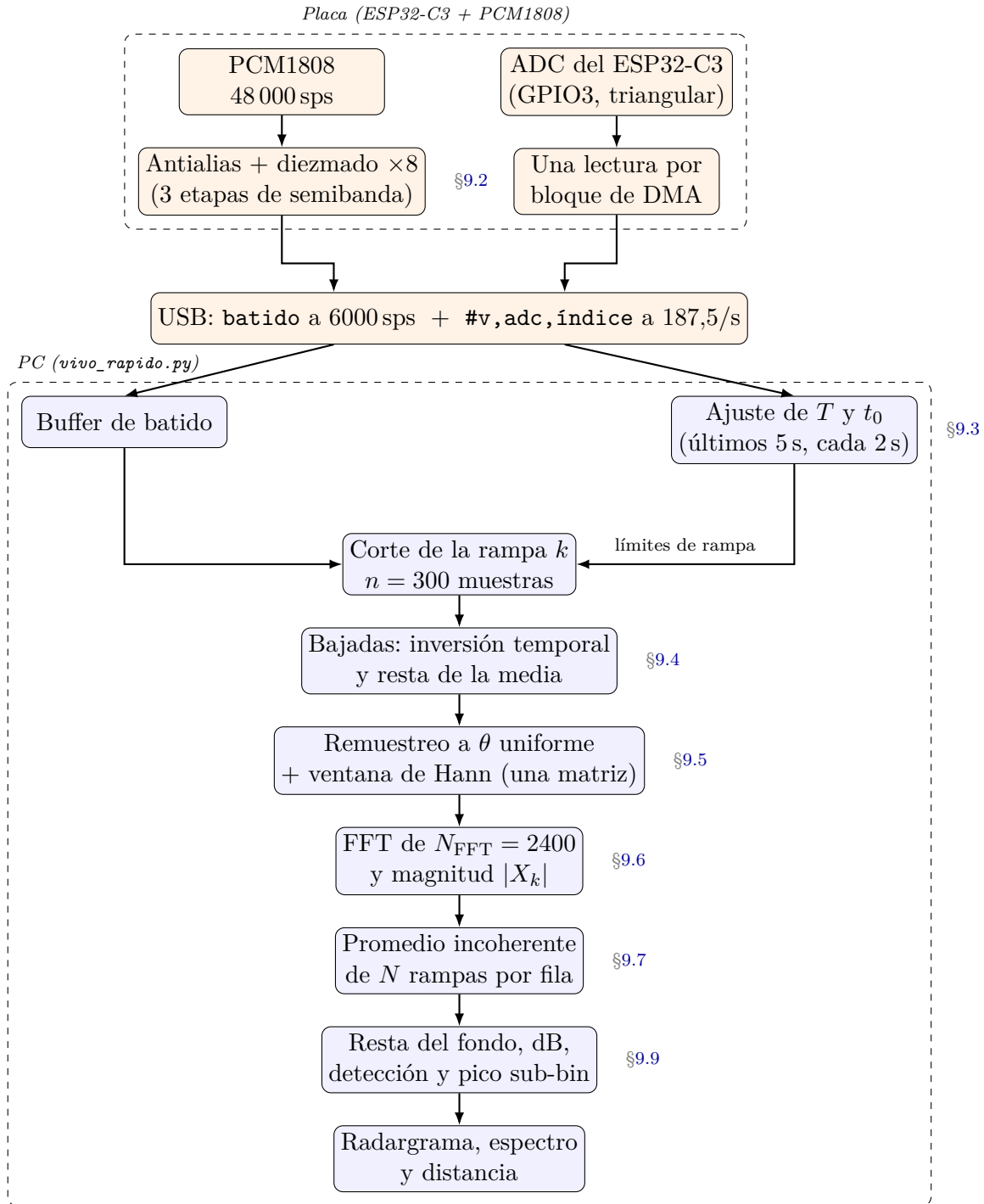
Figura 9.1: Cadena de procesamiento completa. En naranja lo que corre en la placa; en azul lo que corre en la PC. A la derecha de cada bloque, la sección donde se describe.
