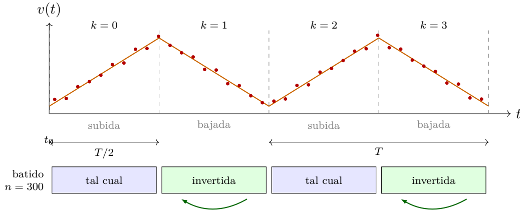
Figura 9.3: Sincronismo reconstruido. Los puntos son las lecturas de la triangular (sólo \sim 19 por período); el triángulo continuo es el modelo ajustado, del que salen los límites de rampa. Cada rampa de batido de 300 muestras se procesa por separado, y las bajadas se invierten en el tiempo.
