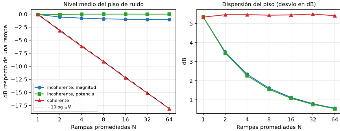
Figura 9.6: Piso de ruido en función de la cantidad de rampas promediadas, sobre 300 realizaciones de ruido puro. Izquierda: nivel medio, referido al de una rampa. Derecha: desvío del piso en dB a lo largo del espectro.
