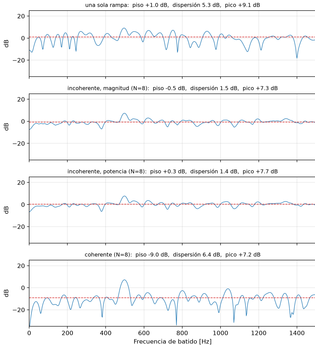
Figura 9.5: Espectro de una fila de N = 8 rampas con un blanco débil en 498 Hz (SNR de -12 dB por muestra en cada rampa), según el criterio de promedio. La línea roja es el piso medio. Una realización; los valores de los títulos varían entre corridas.
