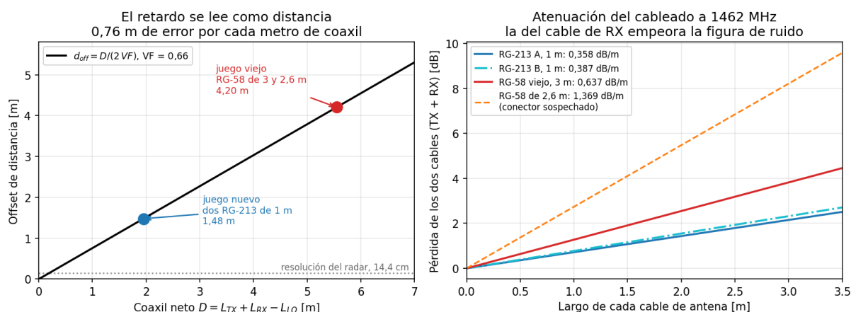
Figura 7.5: Lo que el cableado le cuesta al radar. Izquierda: offset de distancia d_{offset} = D/(2VF) con el VF 0,66 de catálogo, según el coaxil neto D , con los dos juegos de cables marcados. Derecha: pérdida de un par de cables (TX más RX) en el centro de la banda, 1462 MHz, en función del largo de cada uno, con la atenuación por metro medida en cada cable. La recta del RG-58 de 2,6 m es la del cable dañado (Sección 7.6.5), no la de un RG-58.
