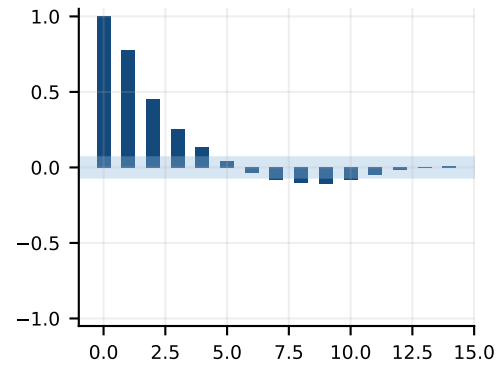
PACF
