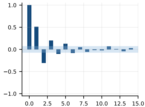
PACF
