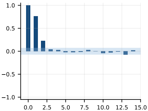
PACF
