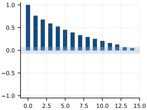
PACF
