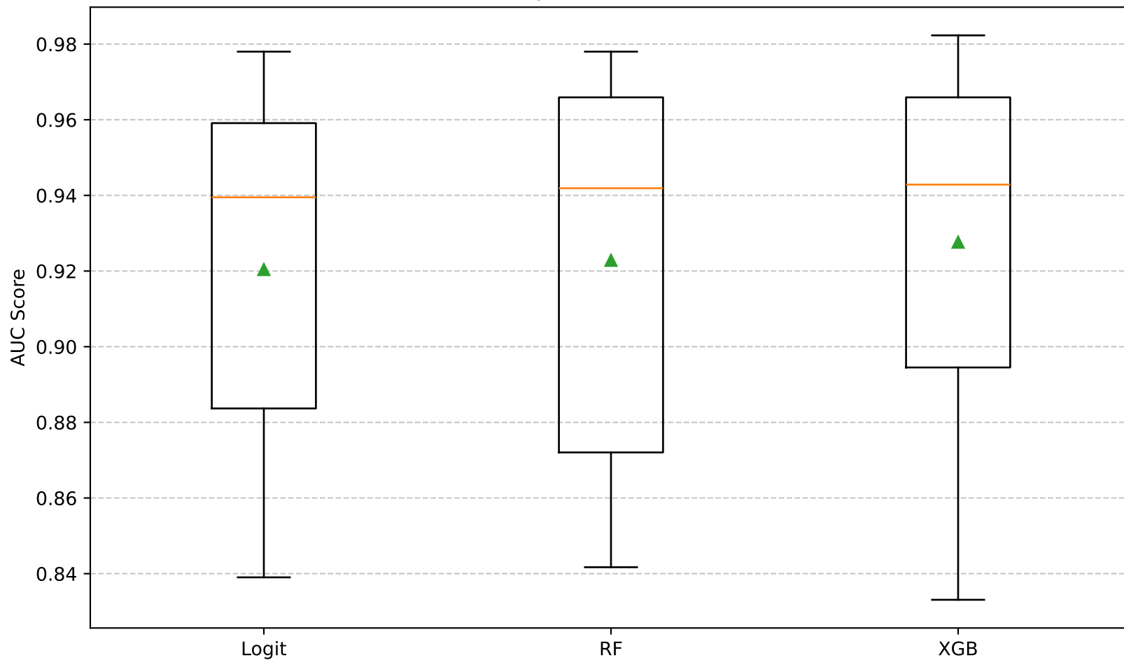
Comparação Estatística de Performance (AUC-ROC) Validação Cruzada 10-fold
