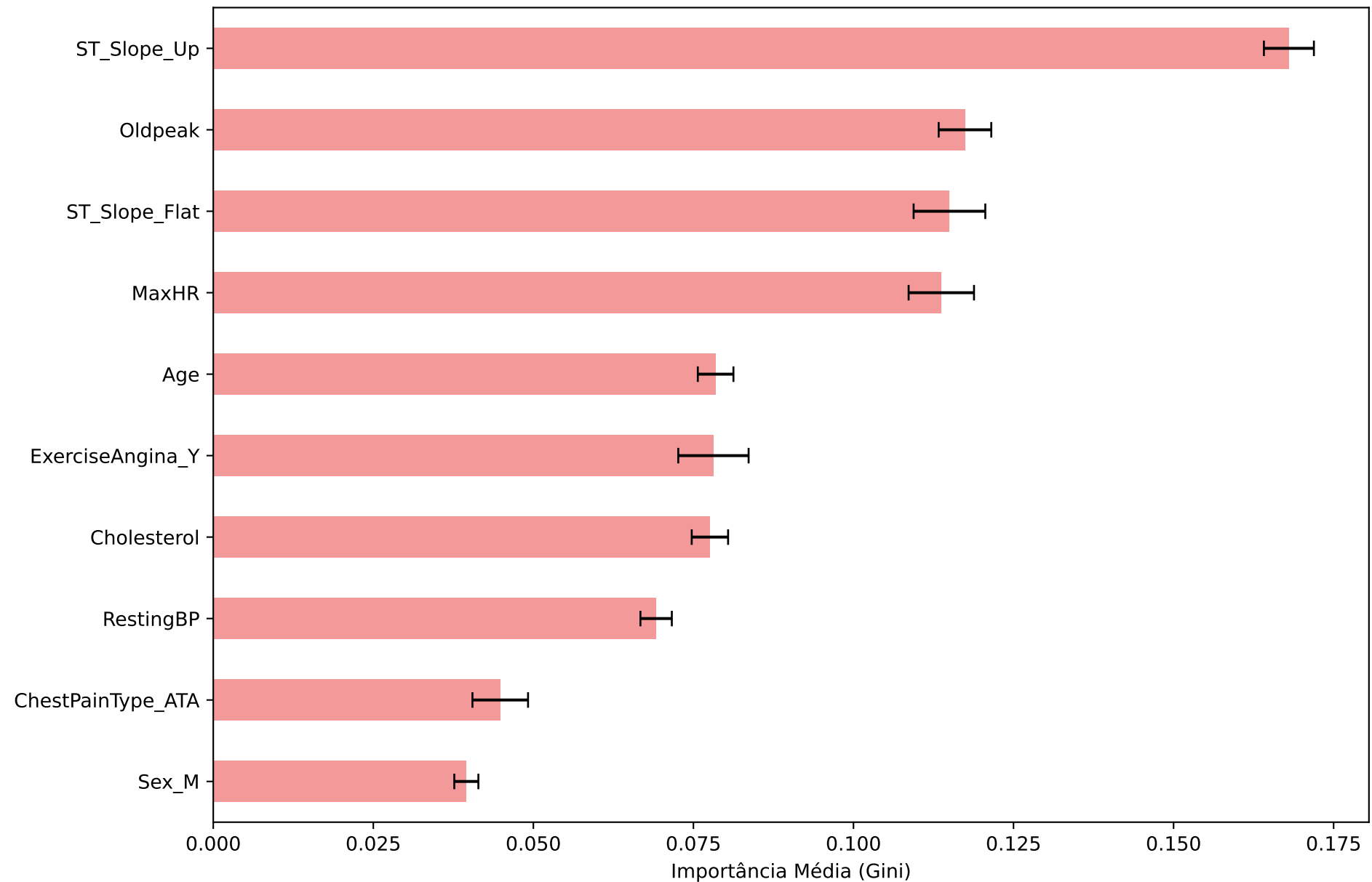
Top 10 Features Mais Importantes - Random Forest (Média \pm Desvio Padrão)
