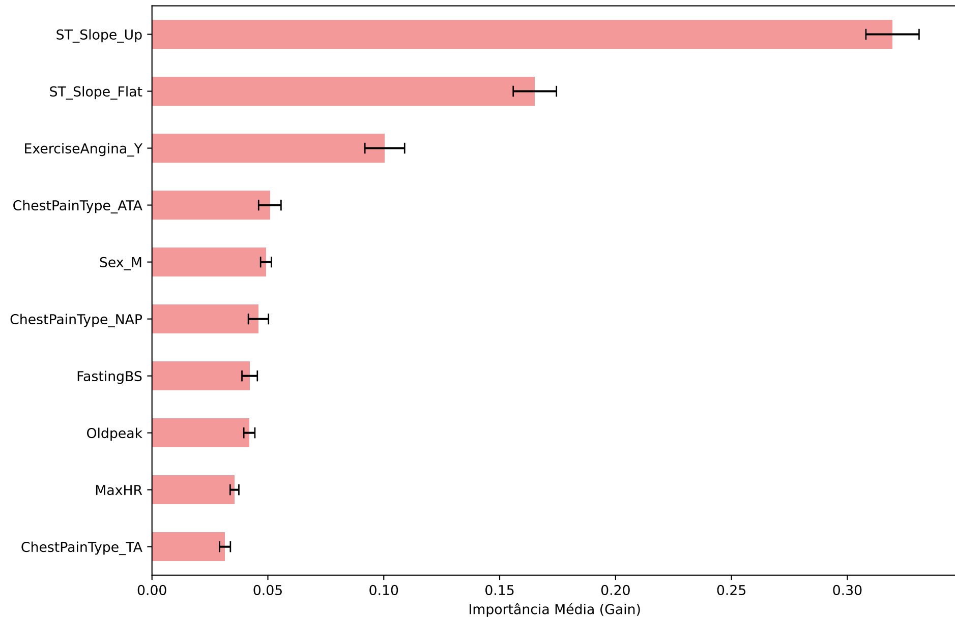
Top 10 Features Mais Importantes - XGBoost (Média \pm Desvio Padrão)
