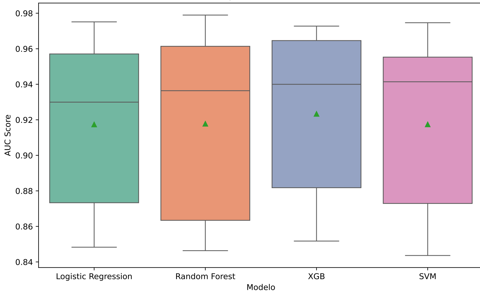
Comparação Estatística de Performance (AUC-ROC) Validação Cruzada 10-fold
