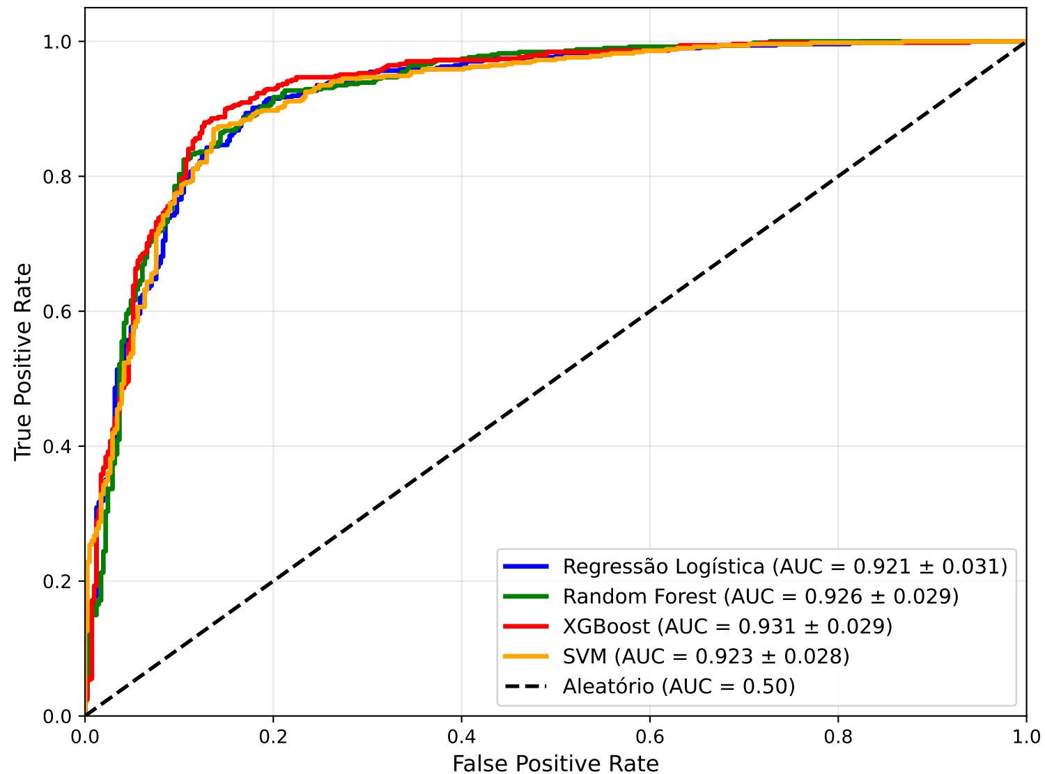
Curva ROC - Validação Cruzada 10-fold Estratificada
