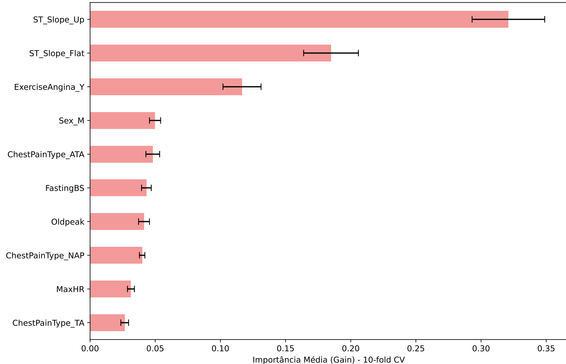
Top 10 Features Mais Importantes - XGBoost (Média \pm Desvio Padrão em Validação Cruzada)
