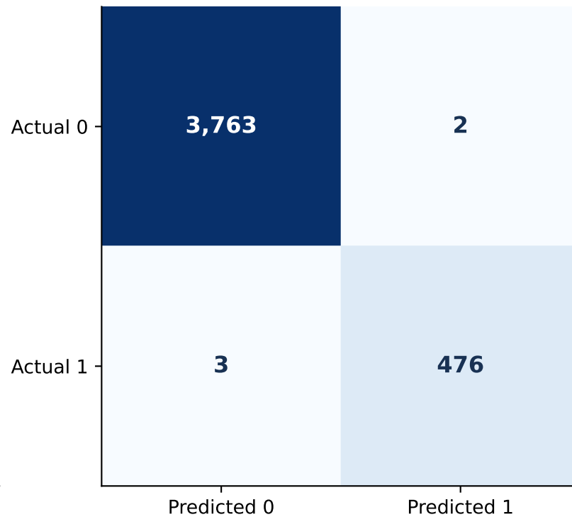
LightGBM F1 = 0.995
