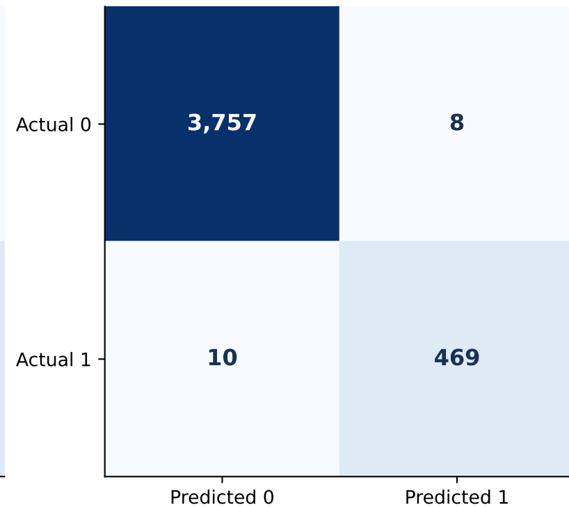
MLP F1 = 0.981
