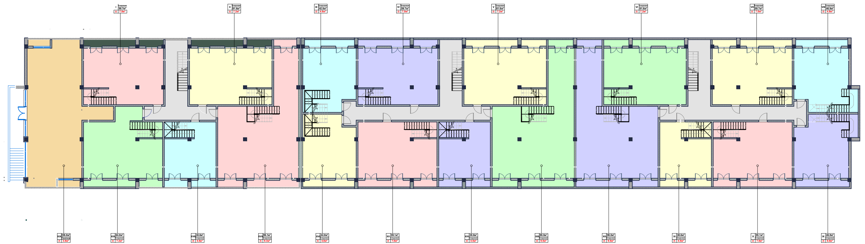
I план подвального этажа на отм: -3,450
