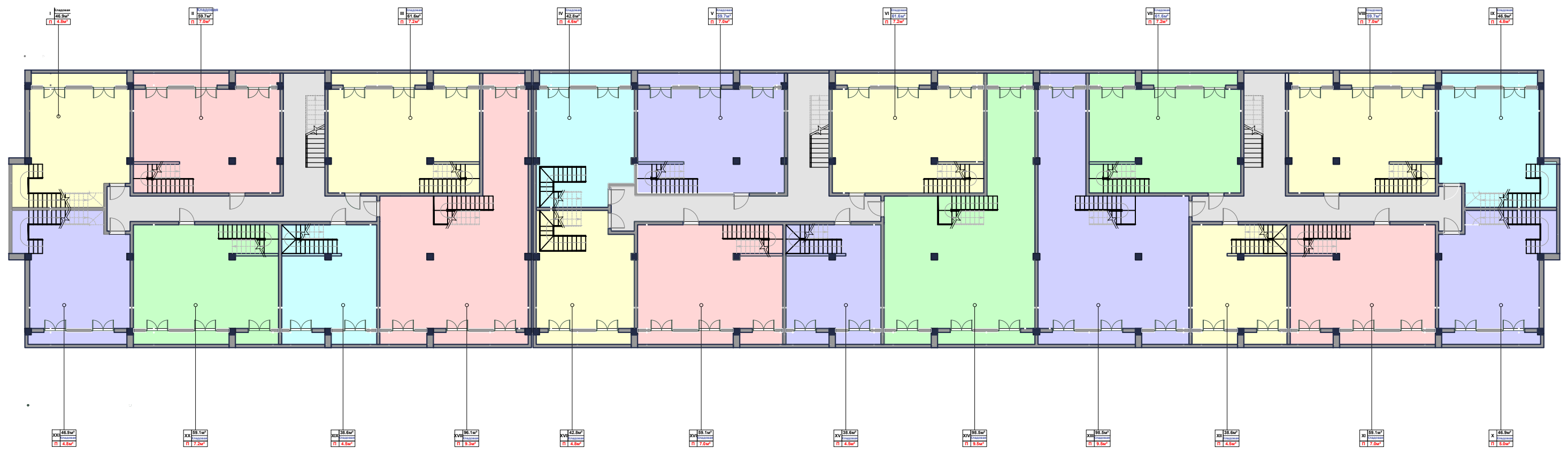
План подвального этажа на отм: -3,450
