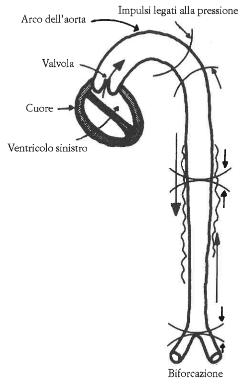
Figura 6: La collisione degli impulsi legati alla pressione che si muovono in senso opposto causa un'interferenza e una vibrazione distruttiva nelle pareti dell'aorta.
