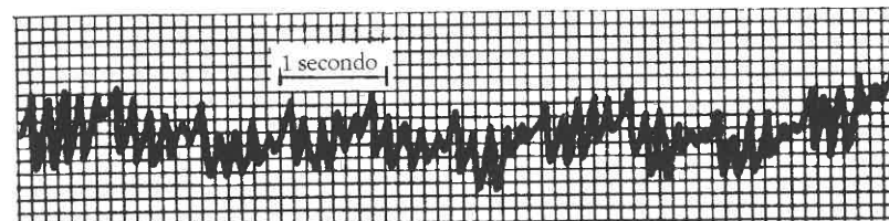
Figura 3: Registrazione di uno stato di profonda meditazione
