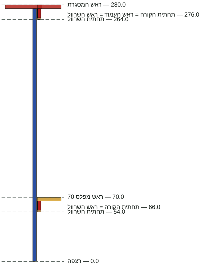
העמוד נגמר בדיוק מתחת למסגרת העליונה. ראש כל שרוול בגובה תחתית הקורה שלו.
