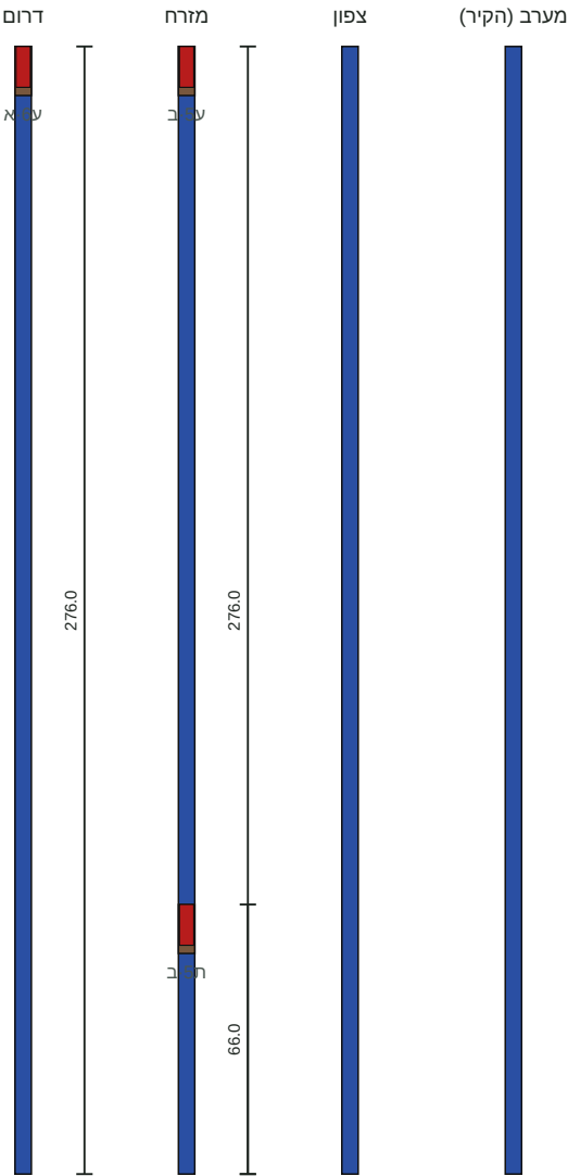
גובה העמוד 276.0 · ראש כל שרול בגובה תחתית הקורה שלו
