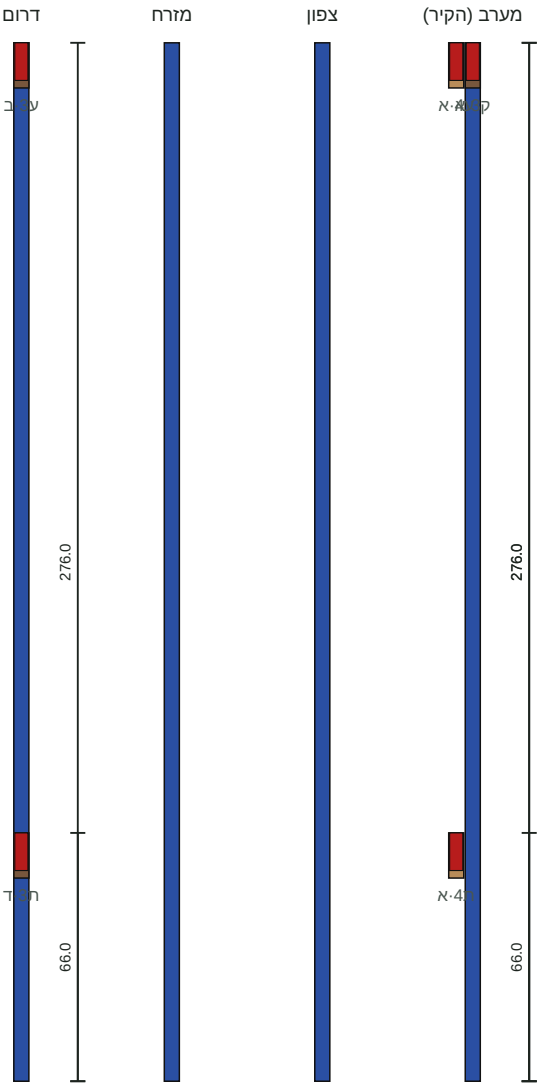
גובה העמוד 276.0 · ראש כל שרוול בגובה תחתית הקורה שלו
