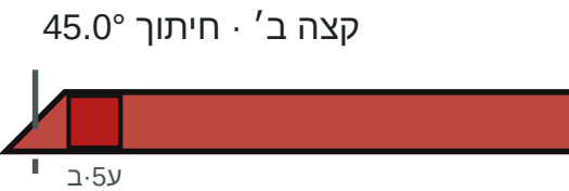
מבט צד — השן מתחת לקורה
