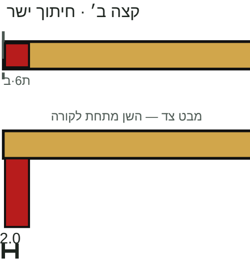
פרט קצה ב' — החיתוך, והשן במרחקה מהקצה על הציר
