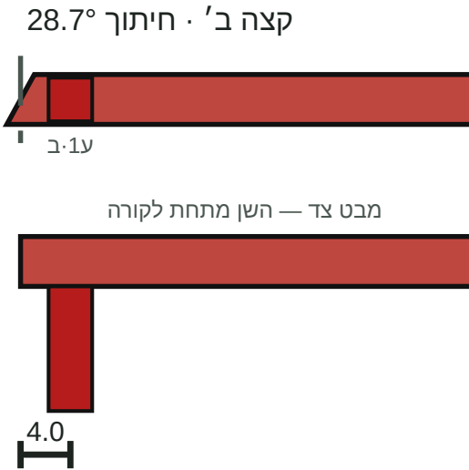
פרט קצה ב' — החיתוך, והשן במרחקה מהקצה על הציר
