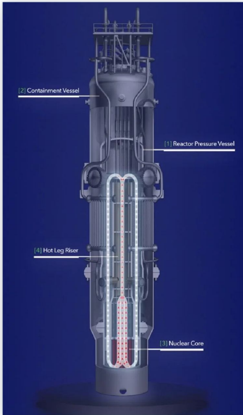
NPM 단면
