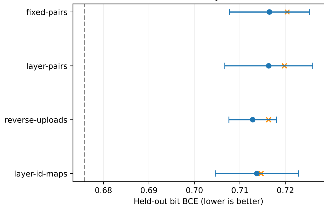
Qwen input
