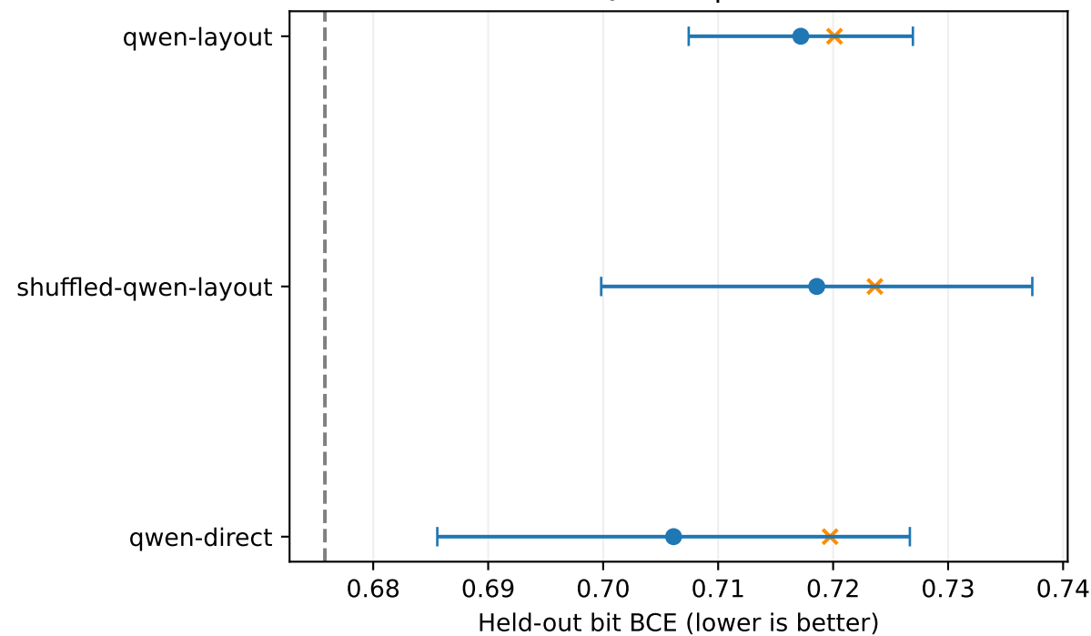
Qwen input
