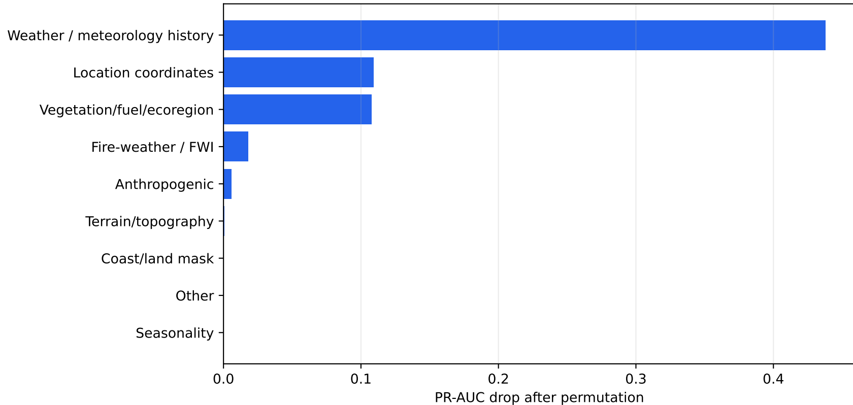
Grouped Permutation Importance
