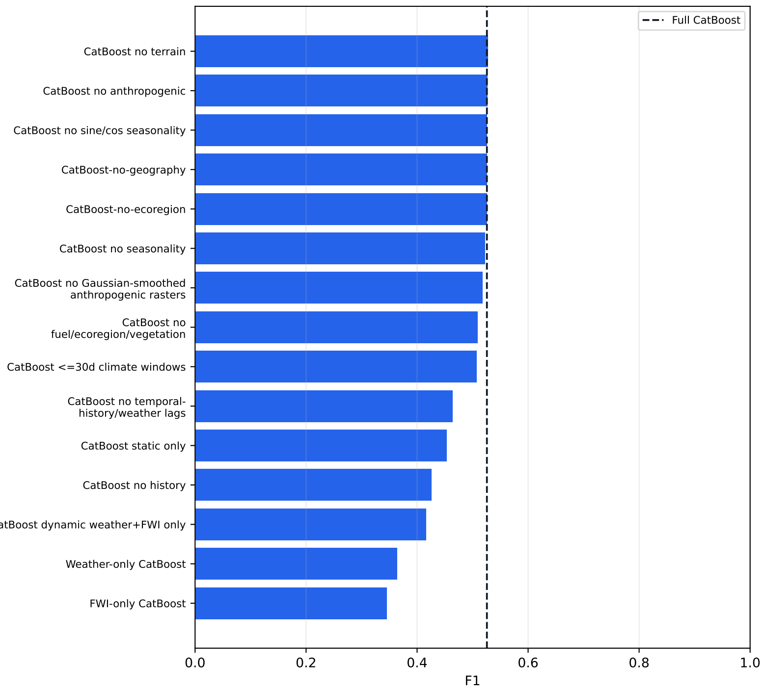
Absolute F1
