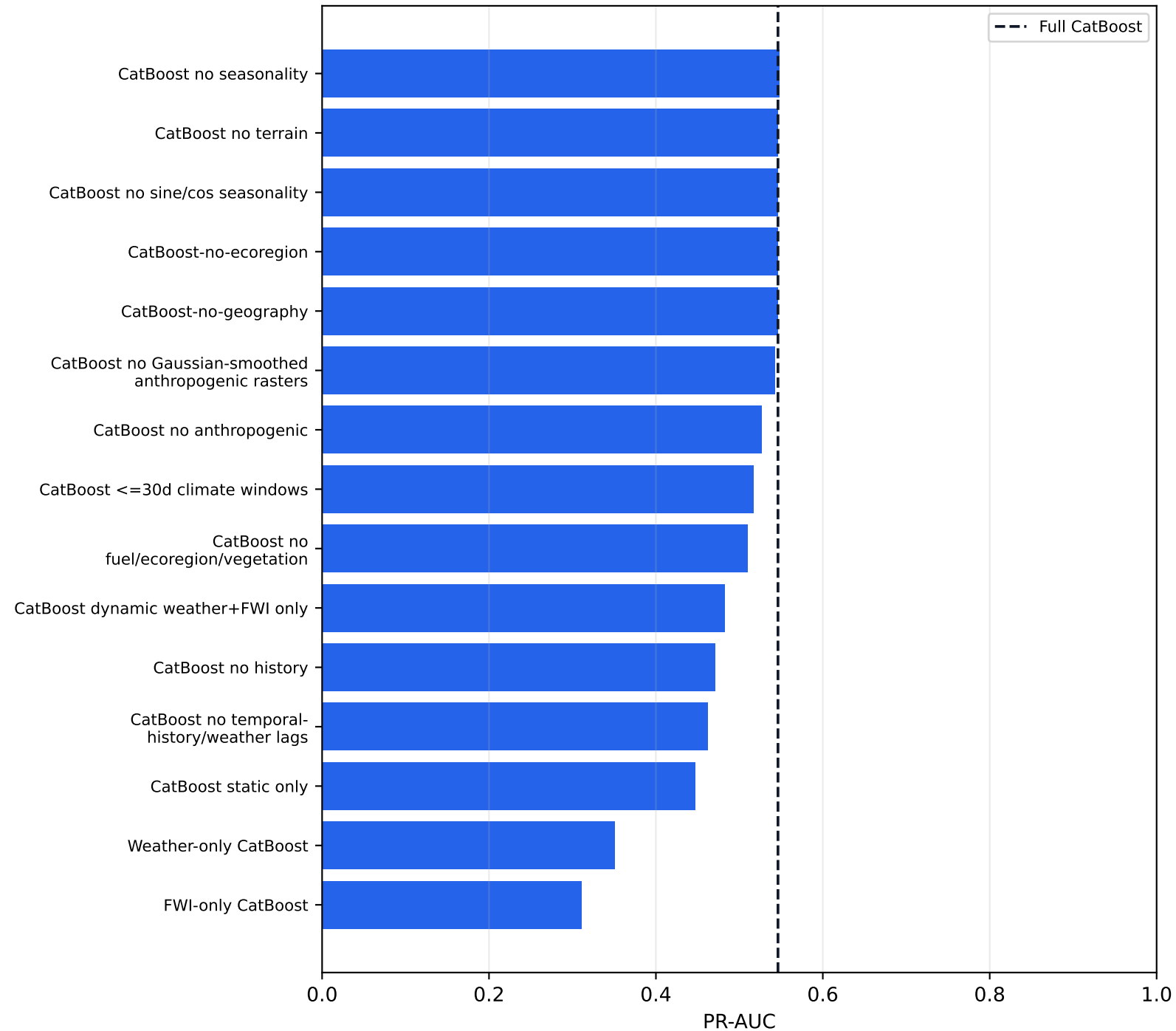
Absolute PR-AUC
