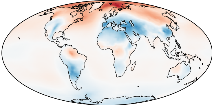
f EC-Earth3-Veg-LR
