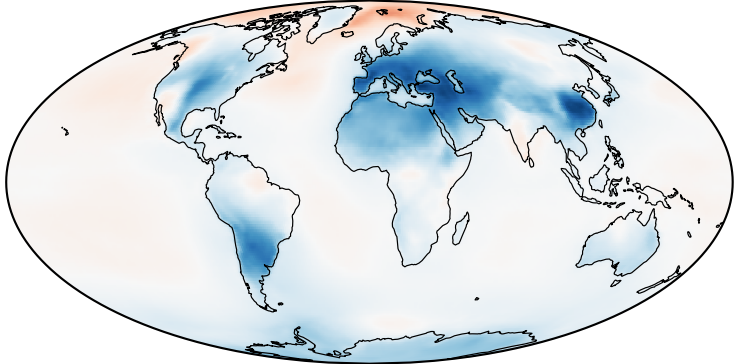
a ERA5
