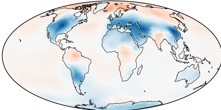
k GISS-E2-1-G-CC
