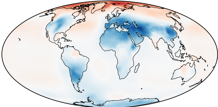
i GFDL-ESM4
