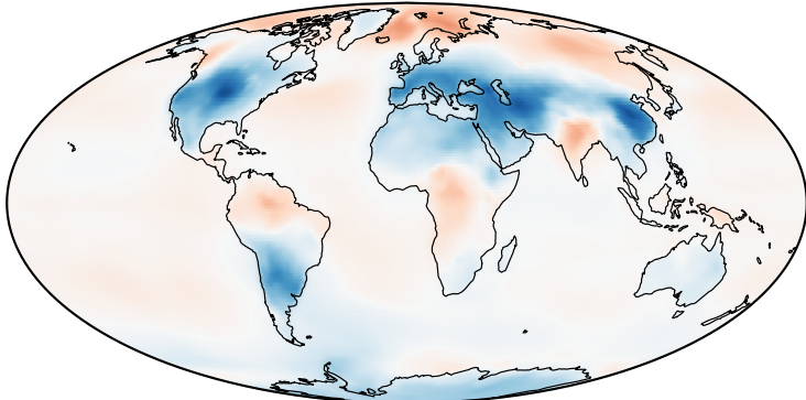
j GISS-E2-1-G
