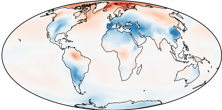
e EC-Earth3-Veg
