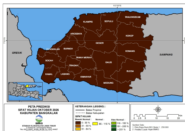
Gambar 4. Peta Prediksi Sifat Hujan Oktober 2026 Bangkalan
