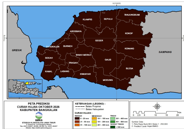
Gambar 3. Peta Prediksi Curah Hujan Oktober 2026 Bangkalan
