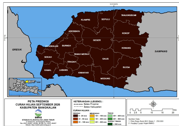
Gambar 1. Peta Prediksi Curah Hujan September 2026 Bangkalan
