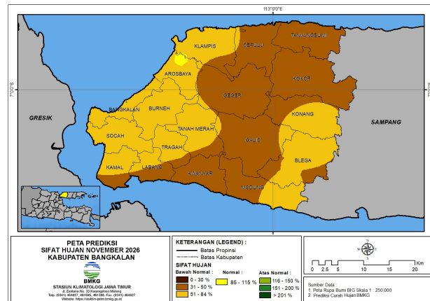
Gambar 6. Peta Prediksi Sifat Hujan November 2026 Bangkalan
