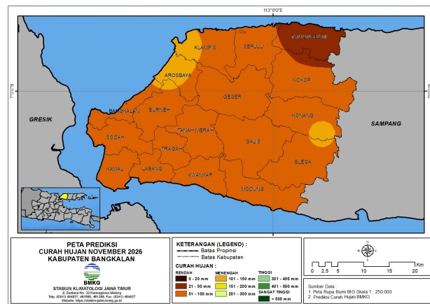
Gambar 5. Peta Prediksi Curah Hujan November 2026 Bangkalan
