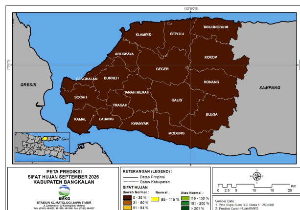
Gambar 2. Peta Prediksi Sifat Hujan September 2026 Bangkalan
