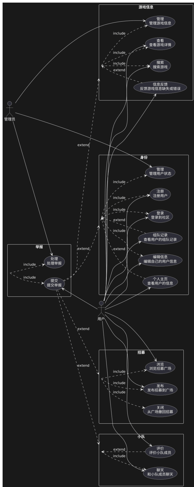
图 1 游戏搭子社区用例模型图
