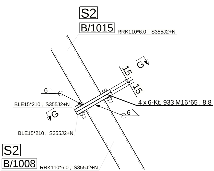
DETAIL 4 : bergseitige Stütze (S2/S3) - Mst: 1:10
