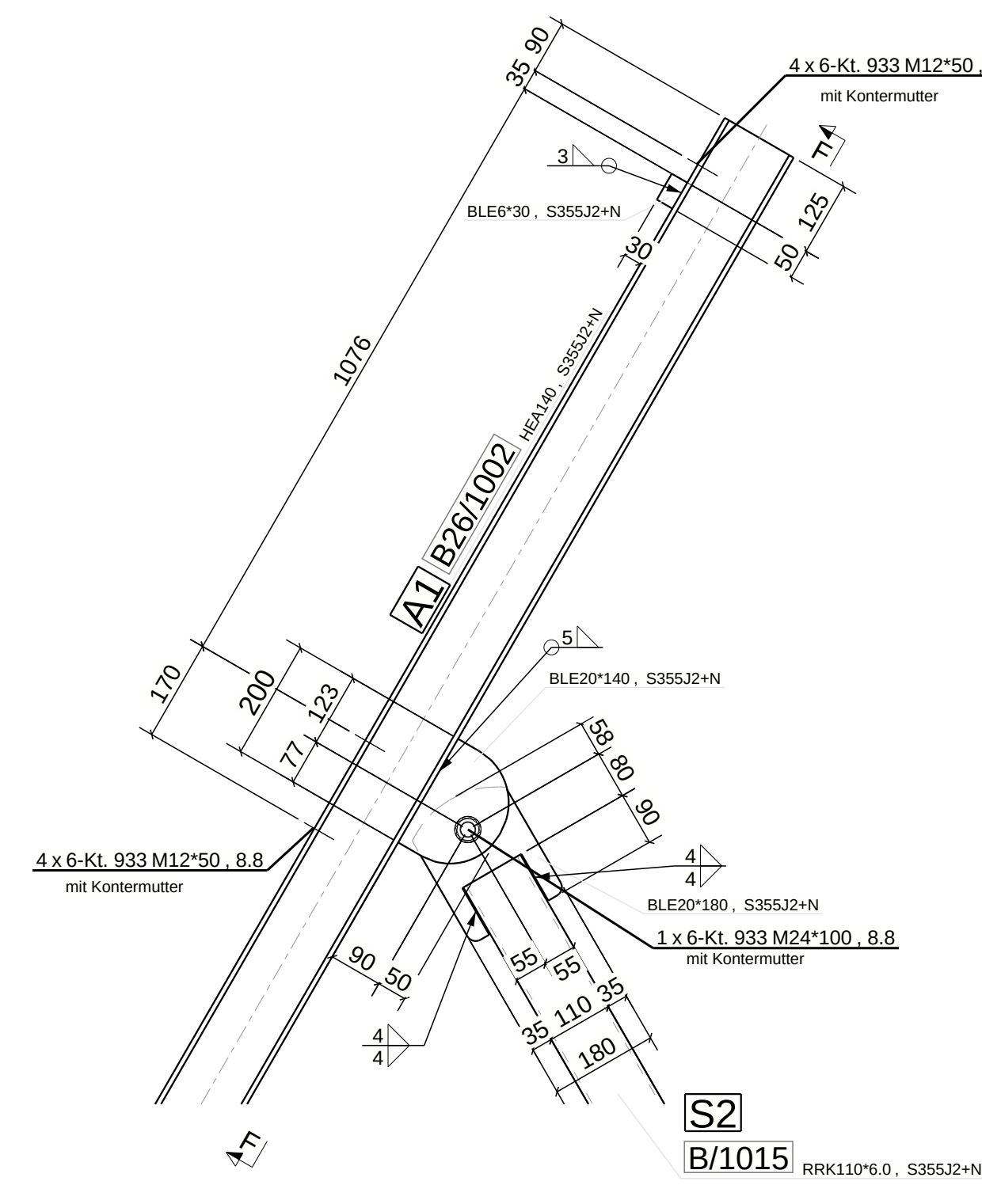
DETAIL 3 : Auflageträger (A1) - Mst: 1:10
