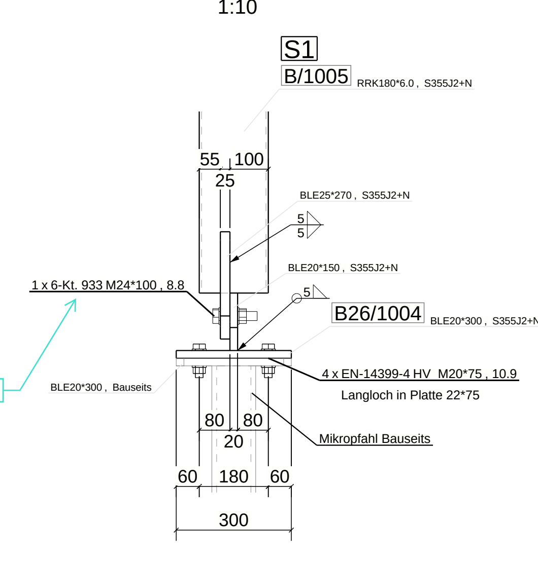
DETAIL 1, Schnitt B - B : talseitiger Stützenfuss (S1/S4)
