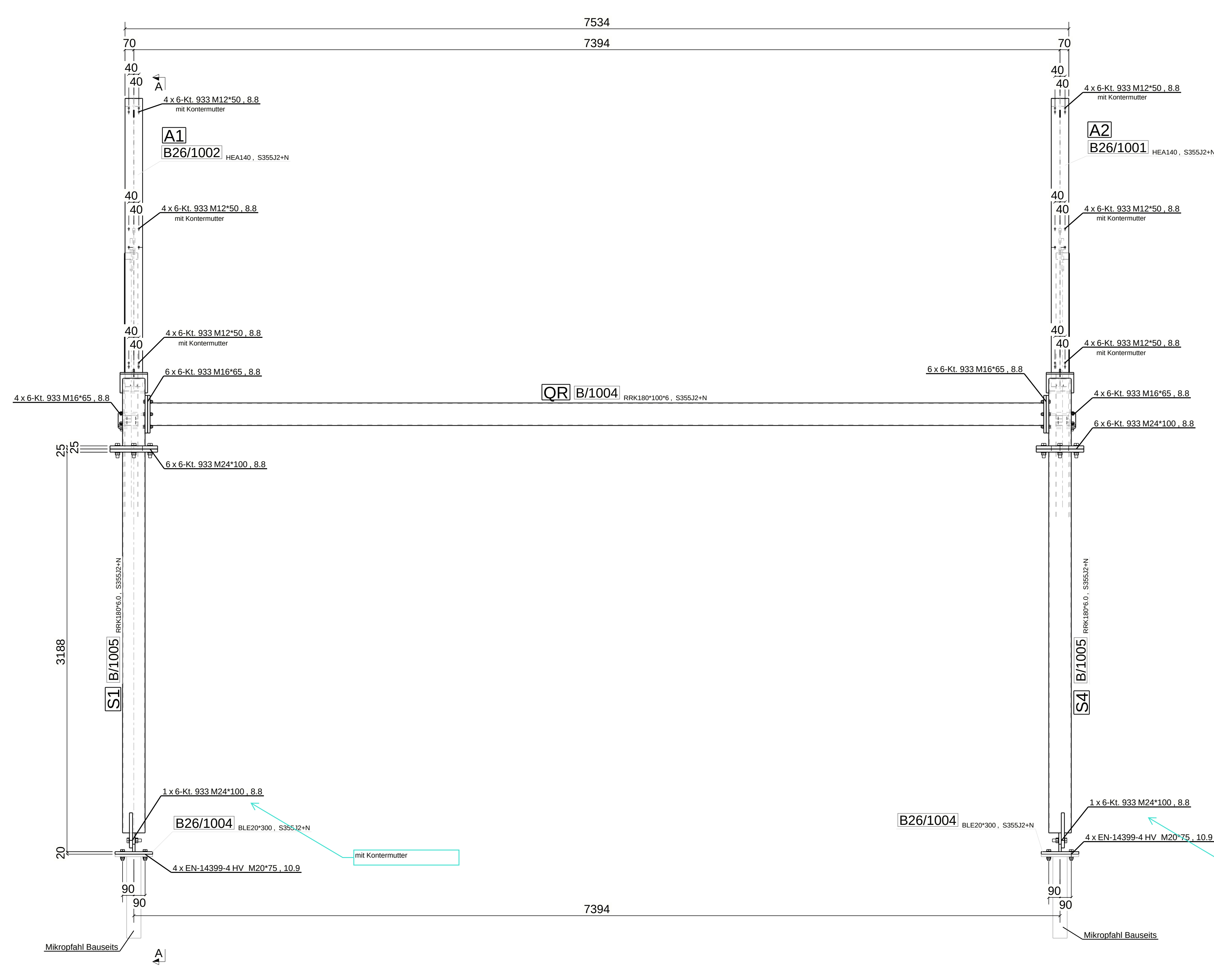
Ansicht: Primärkonstruktion Typ B - 2026 1:20
