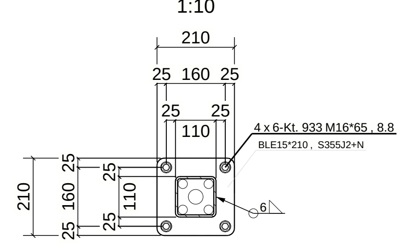
DETAIL 4, Schnitt G - G : bergseitige Stütze (S2/S3)
