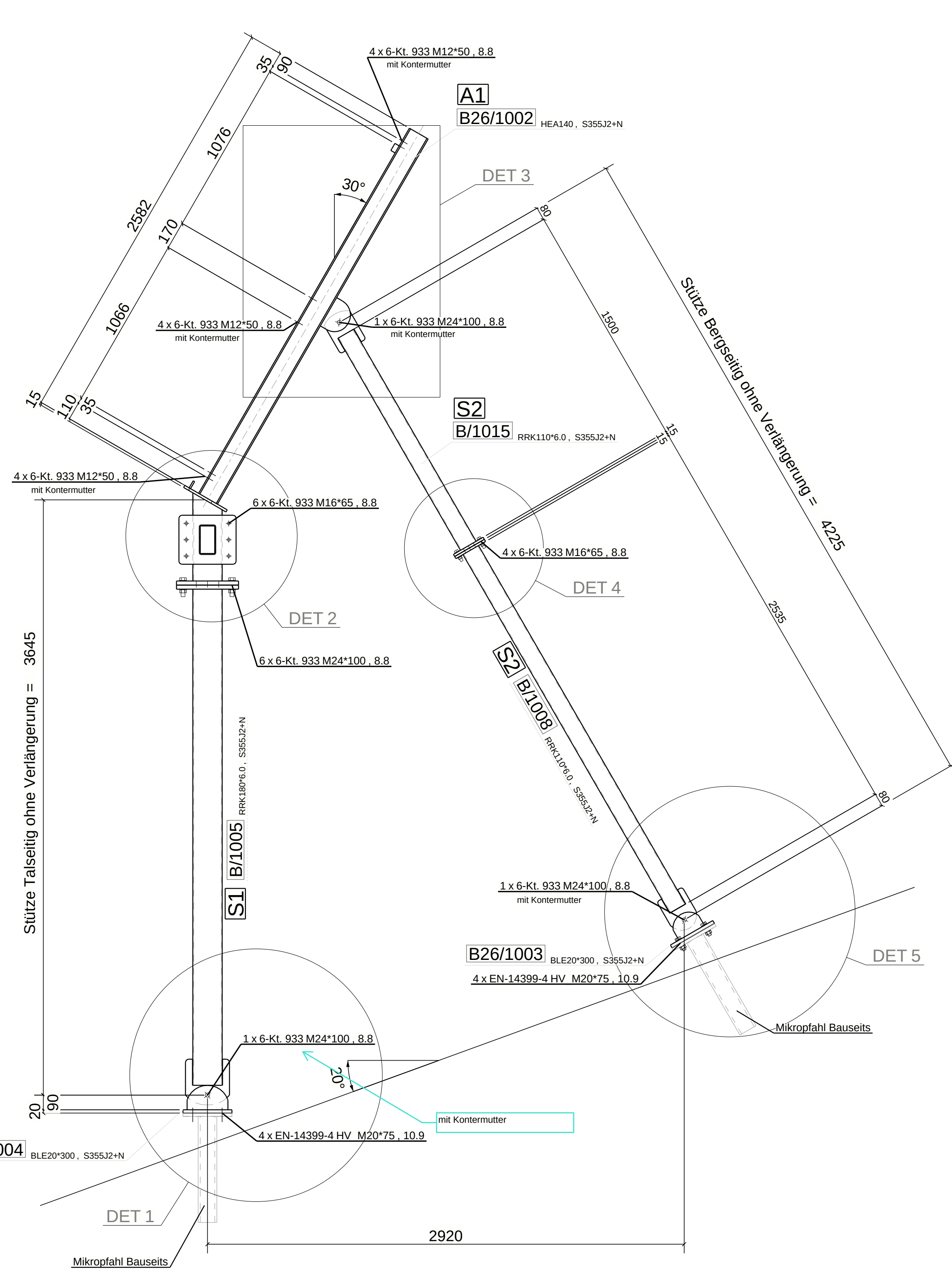
A - A Schnitt: Primärkonstruktion Typ B - 2026 1:20
