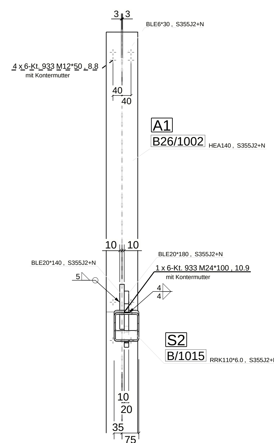
DETAIL 3, Schnitt F - F : Auflageträger (A1) 1:10
