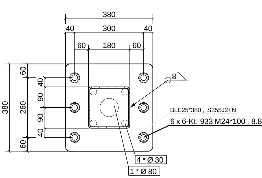
DETAIL 2, Schnitt E - E : talseitige Stütze (S1/S4) 1:10
