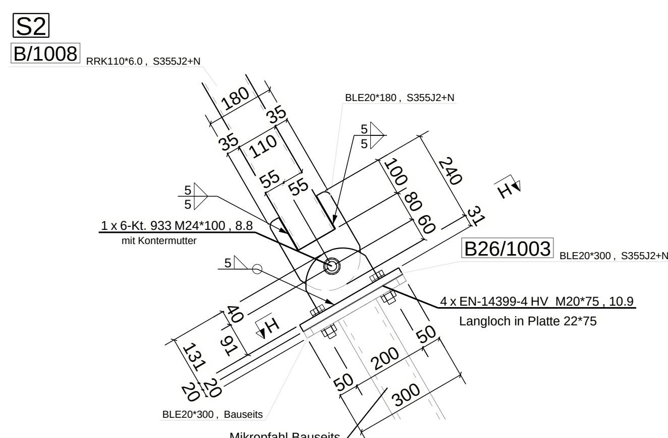
DETAIL 5, Schnitt H - H 3: bergseitiger Stützenfuss (S2/S3)
