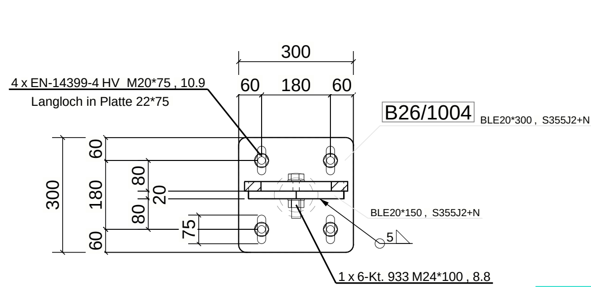
DETAIL 1, Schnitt C - C : talseitiger Stützenfuss (S1/S4) 1:10
