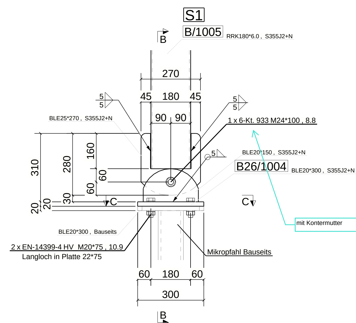
DETAIL 1: talseitiger Stützenfuss (S1/S4) - Mst: 1:10
