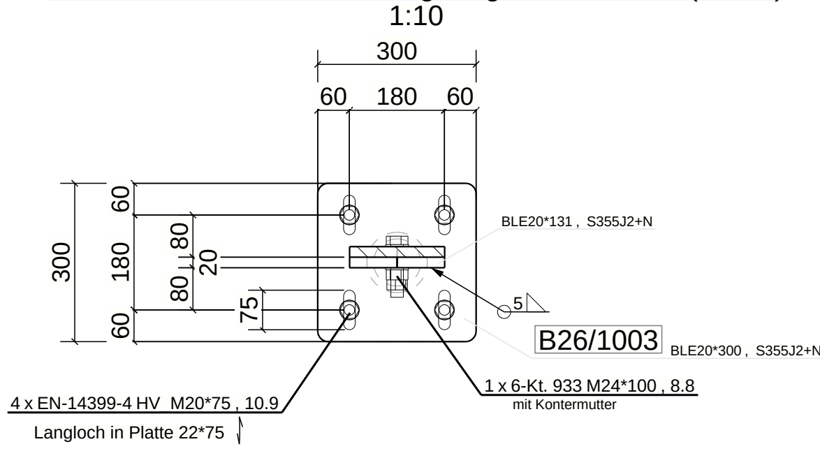
DETAIL 5, Schnitt H - H 3: bergseitiger Stützenfuss (S2/S3)
