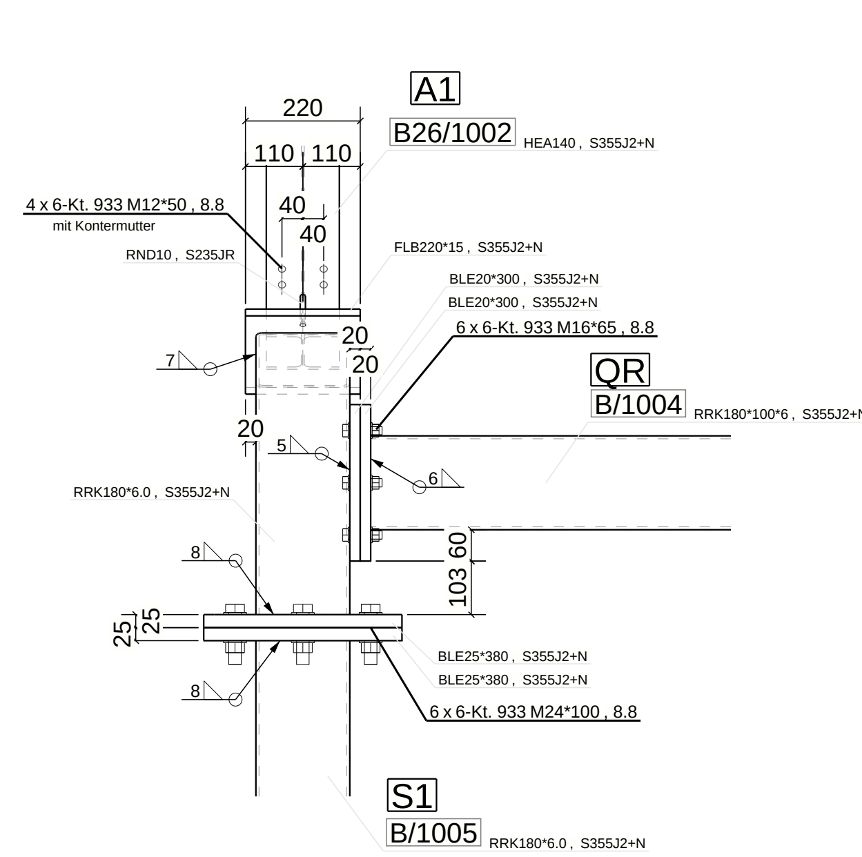
DETAIL 2, Schnitt D - D : talseitige Stütze (S1/S4) 1:10
