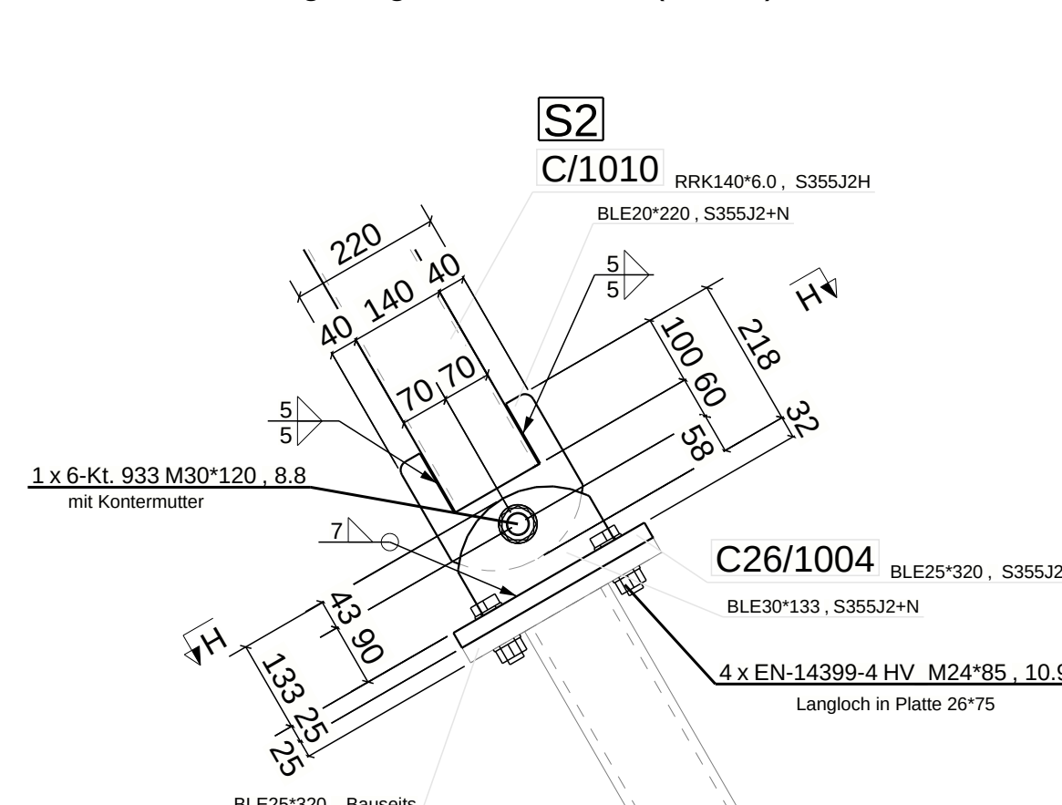
DETAIL 5 : bergseitiger Stützenfuss (S2/S3) - Mst: 1:10
