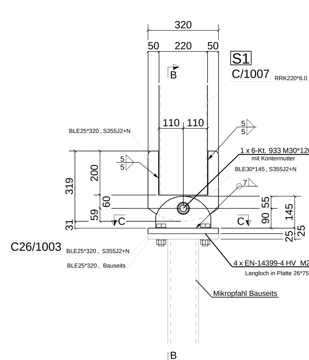
DETAIL 1: talseitiger Stützenfuss (S1/S4) - Mst: 1:10
