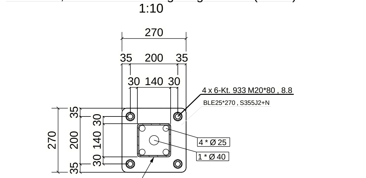
DETAIL 4, Schnitt G - G : bergseitige Stütze (S2/S3)
