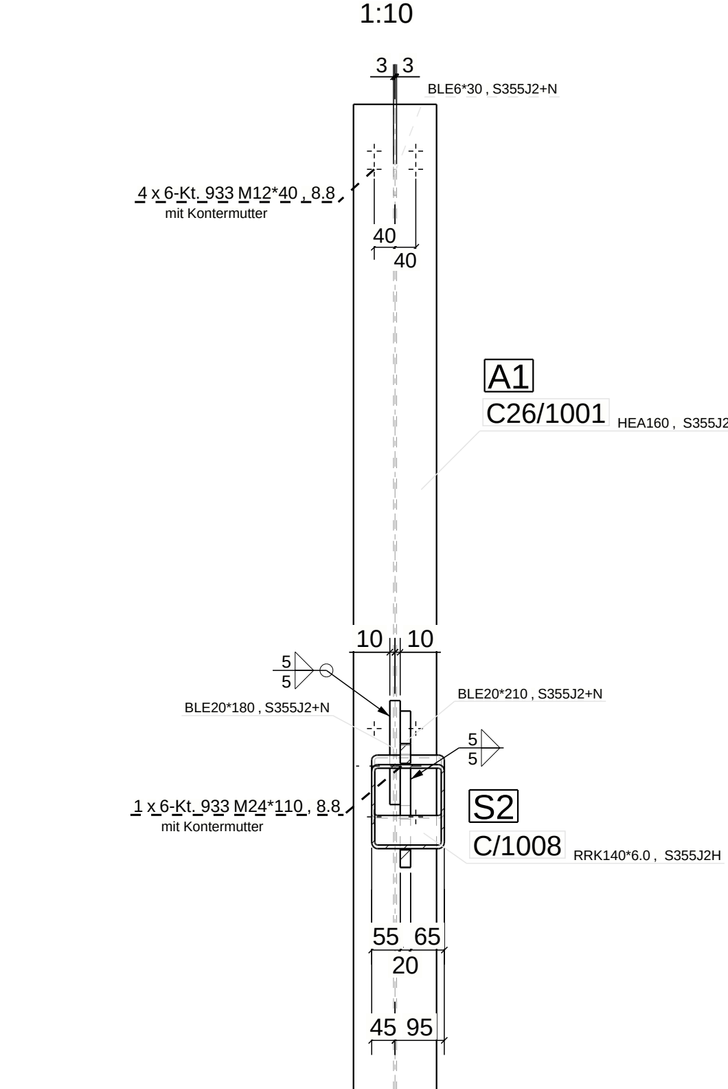
DETAIL 3, Schnitt F - F : Auflageträger (A1)
