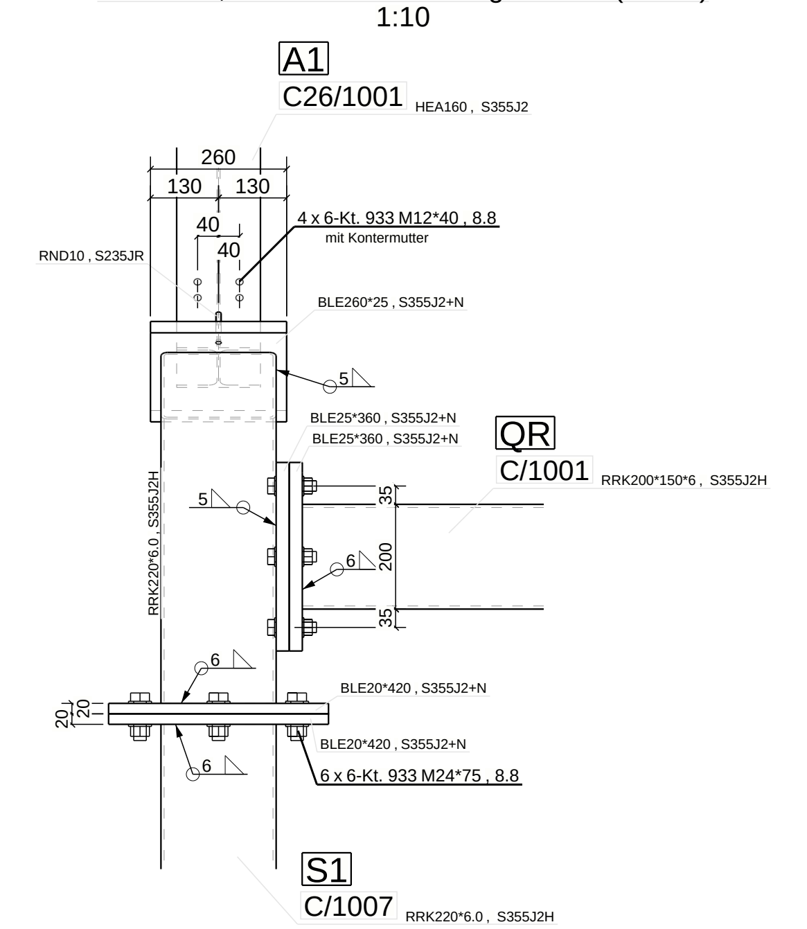
DETAIL 2, Schnitt D - D : talseitige Stütze (S1/S4)
