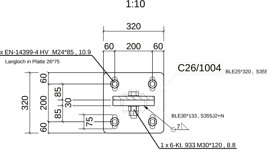
DETAIL 5, Schnitt H - H : bergseitiger Stützenfuss (S2/S3)
