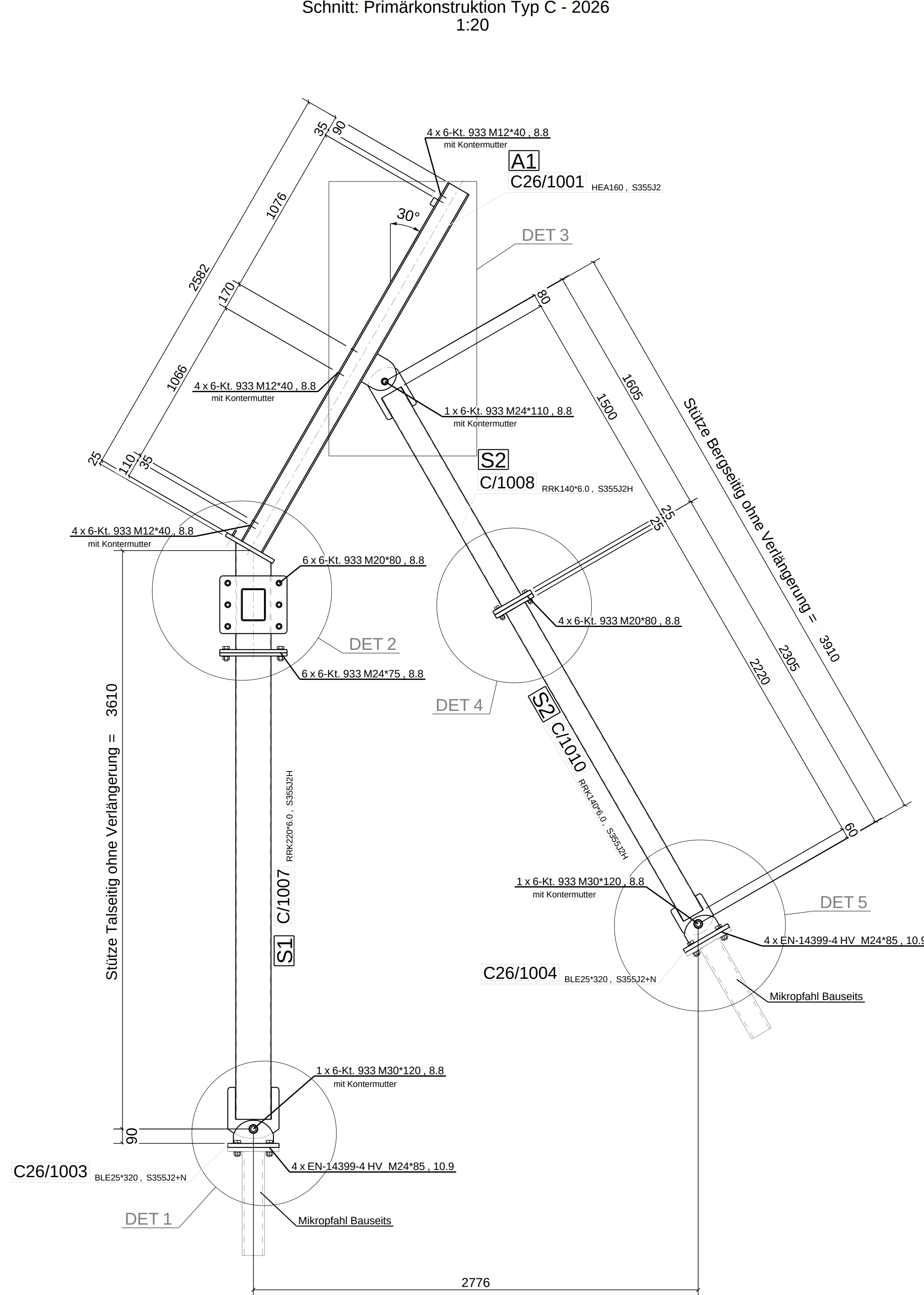
A - A Schnitt: Primärkonstruktion Typ C - 2026
