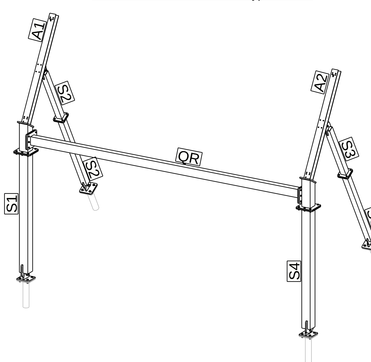
Isometrie Primärkonstruktion Typ C - 2026
