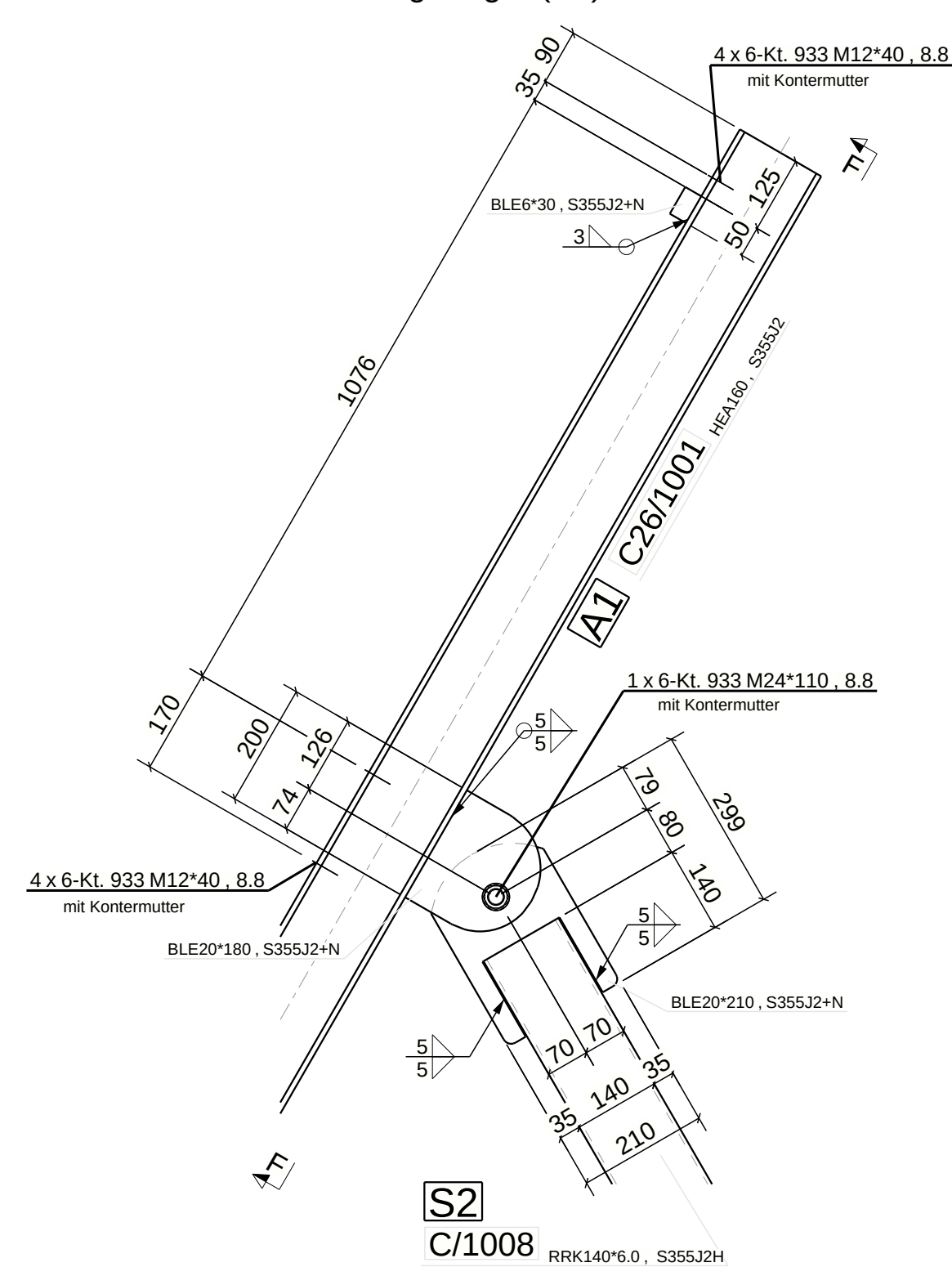
DETAIL 3 : Auflageträger (A1) - Mst: 1:10
