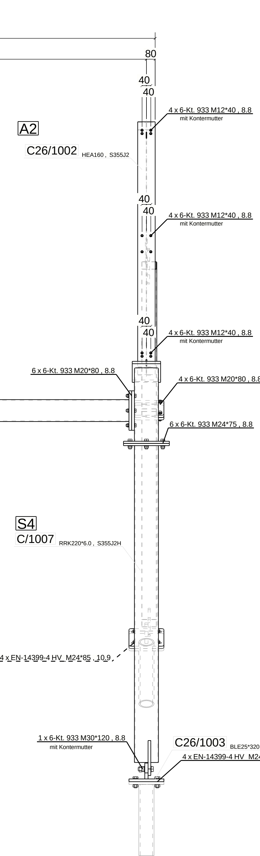
Ansicht: Primärkonstruktion Typ C - 2026
