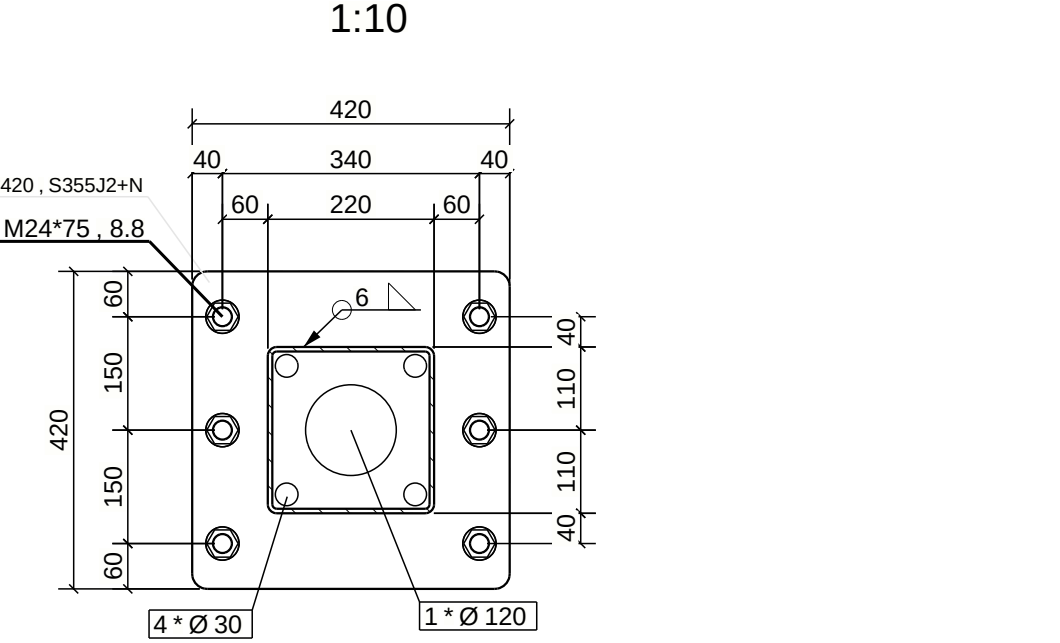
DETAIL 2, Schnitt E - E : talseitige Stütze (S1/S4)
