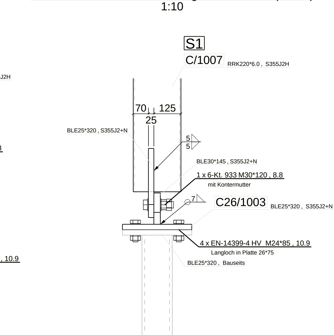
DETAIL 1, Schnitt B - B : talseitiger Stützenfuss (S1/S4)
