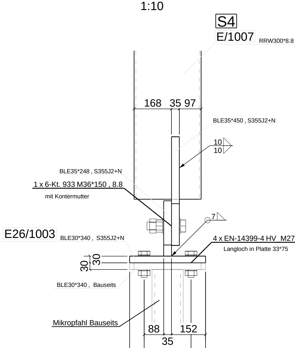
DETAIL 1, Schnitt B - B : talseitiger Stützenfuss (S1/S4)
