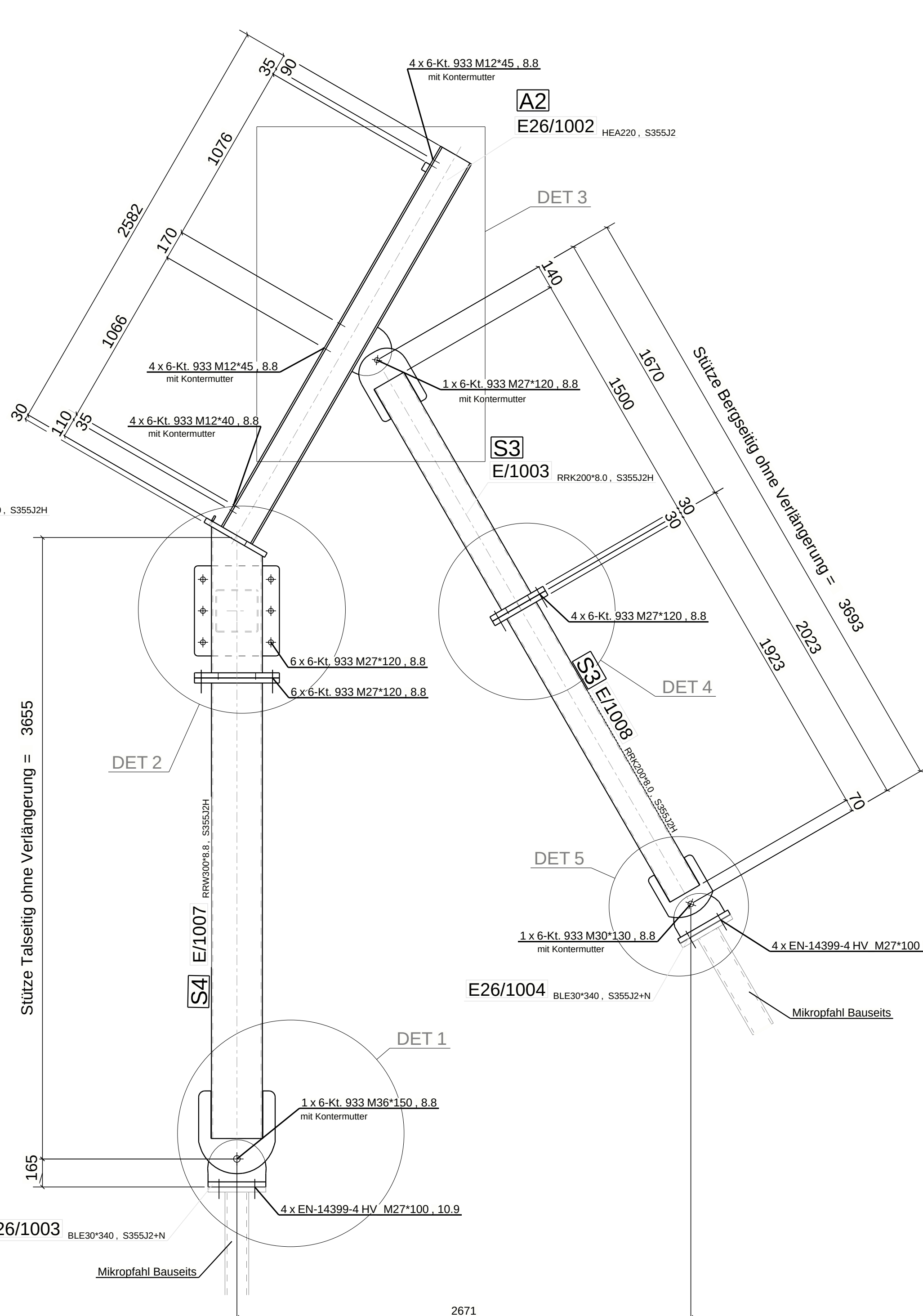
A - A Schnitt: Primärkonstruktion Typ E - 2026
