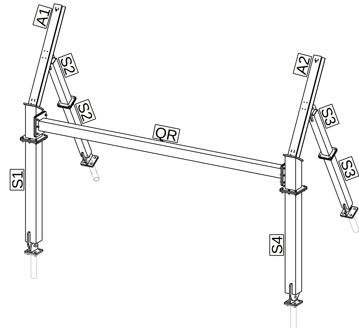
Isometrie Primärkonstruktion Typ E - 2026
