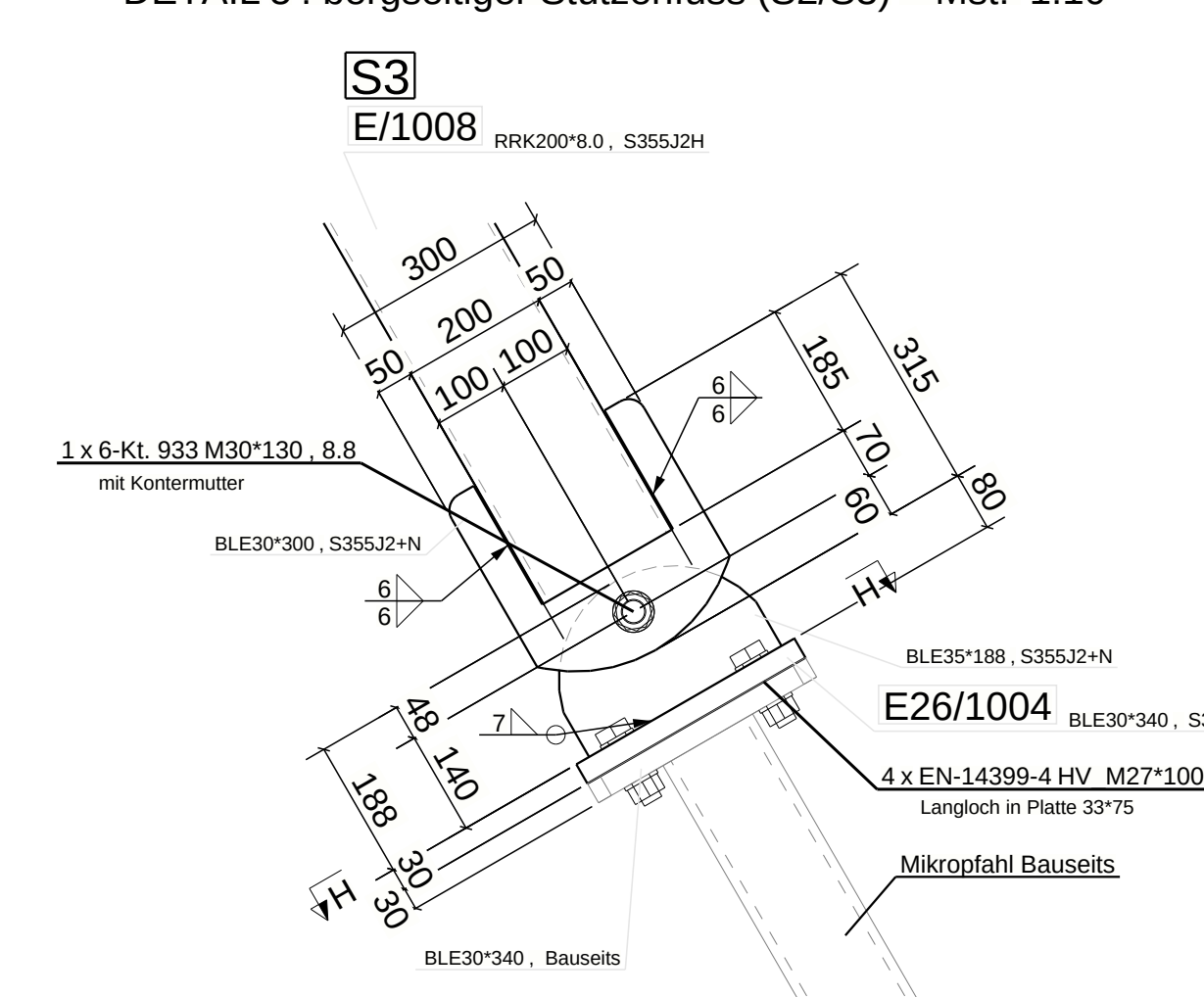
DETAIL 5 : bergseitiger Stützenfuss (S2/S3) - Mst: 1:10
