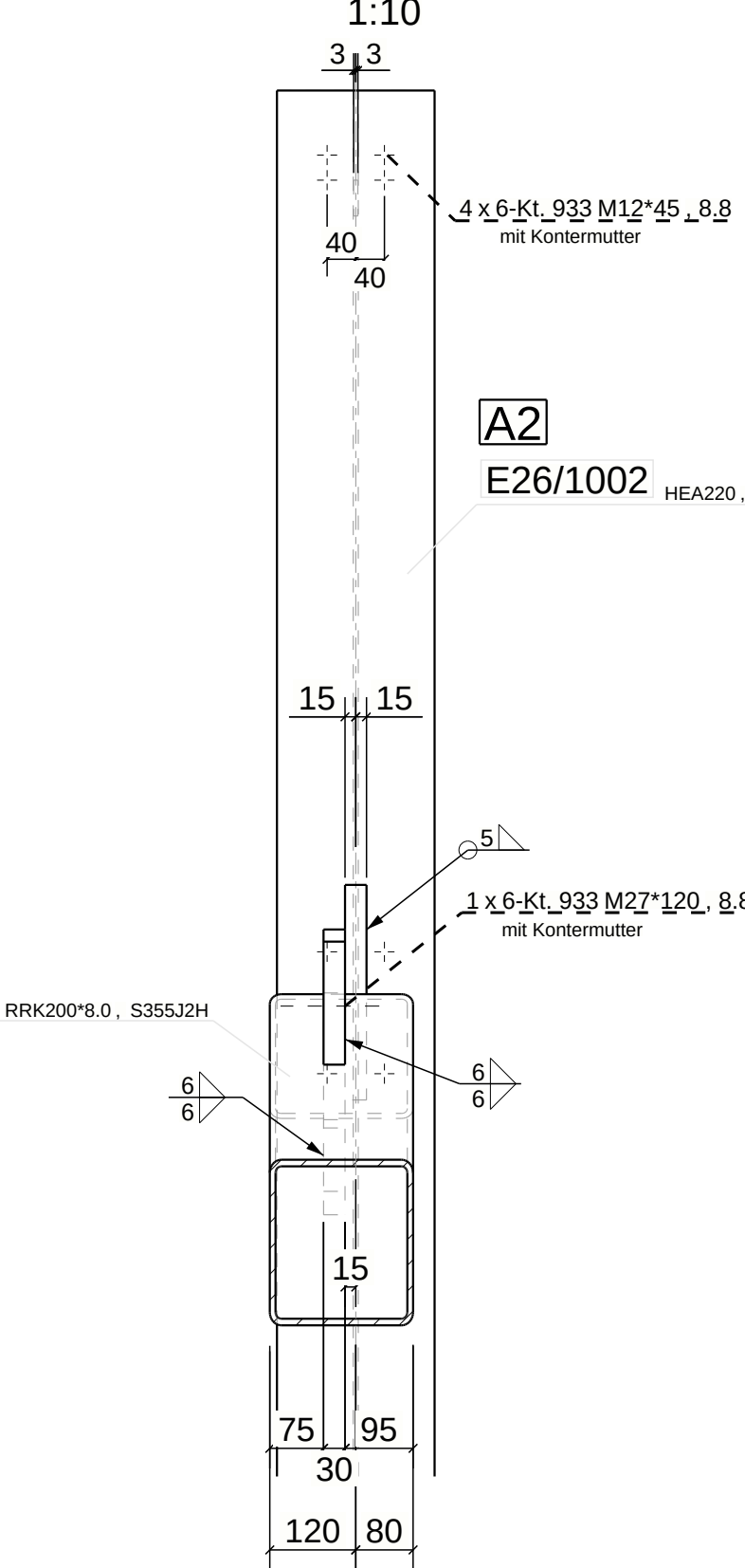
DETAIL 2, Schnitt D - D : talseitige Stütze (S1/S4)
