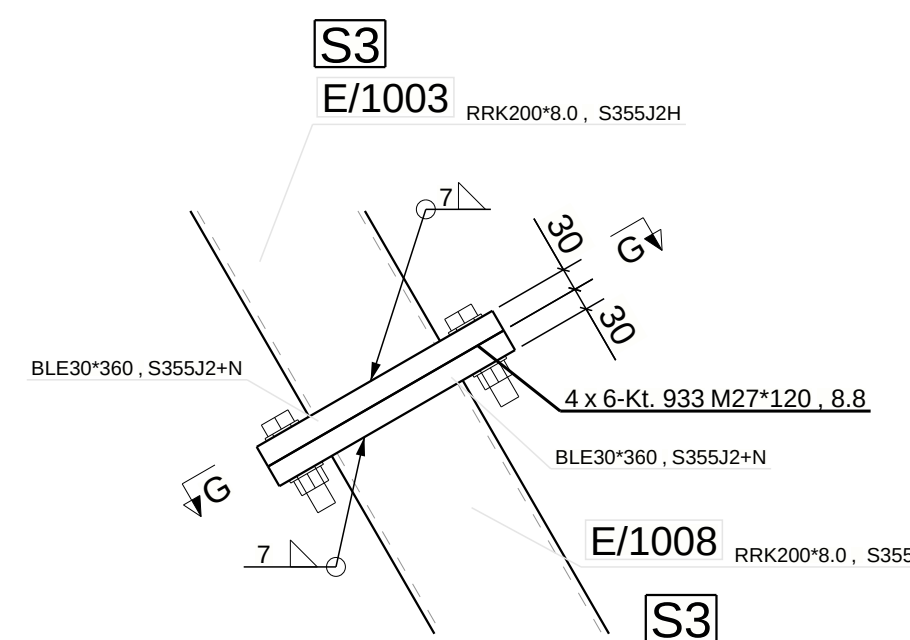
DETAIL 4 : bergseitige Stütze (S2/S3) - Mst: 1:10
