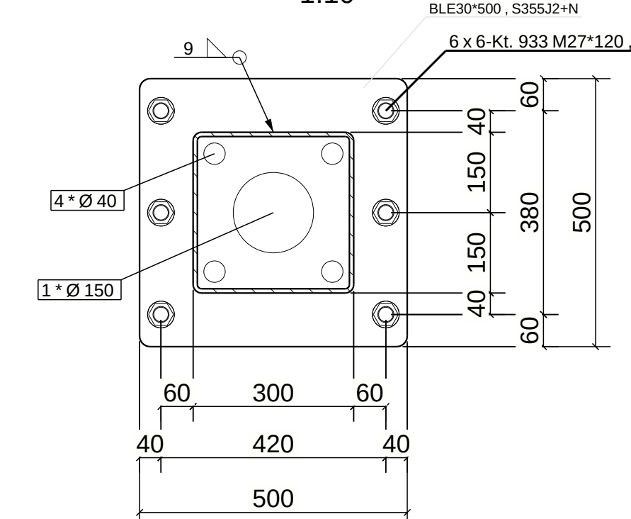
DETAIL 1: talseitiger Stützenfuss (S1/S4) - Mst: 1:10
