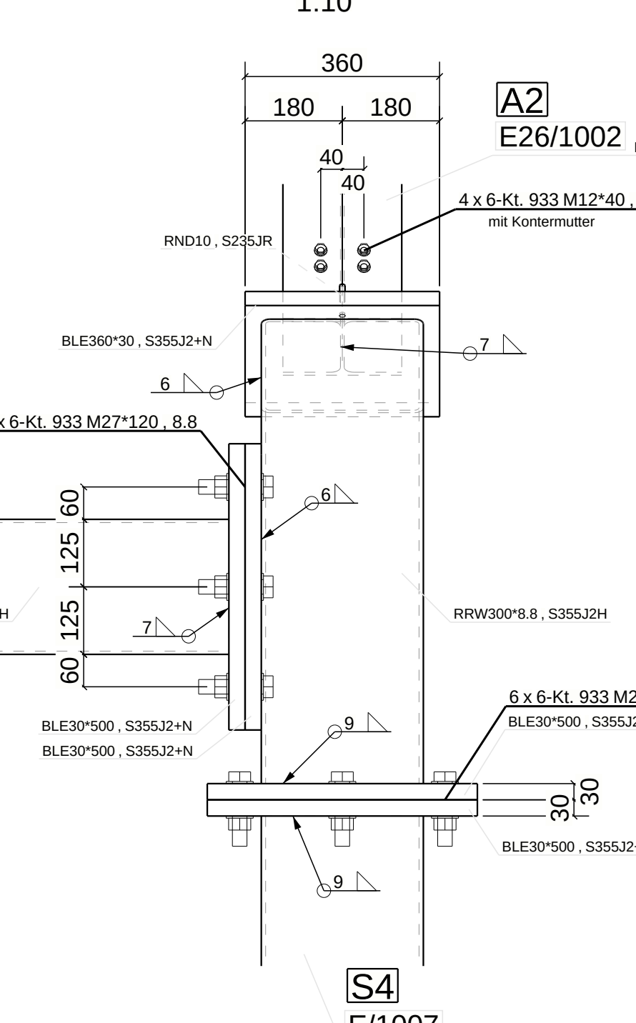
DETAIL 2, Schnitt D - D : talseitige Stütze (S1/S4)
