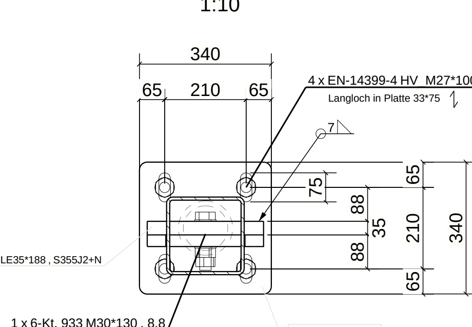
DETAIL 5, Schnitt H - H 3: bergseitiger Stützenfuss (S2/S3)
