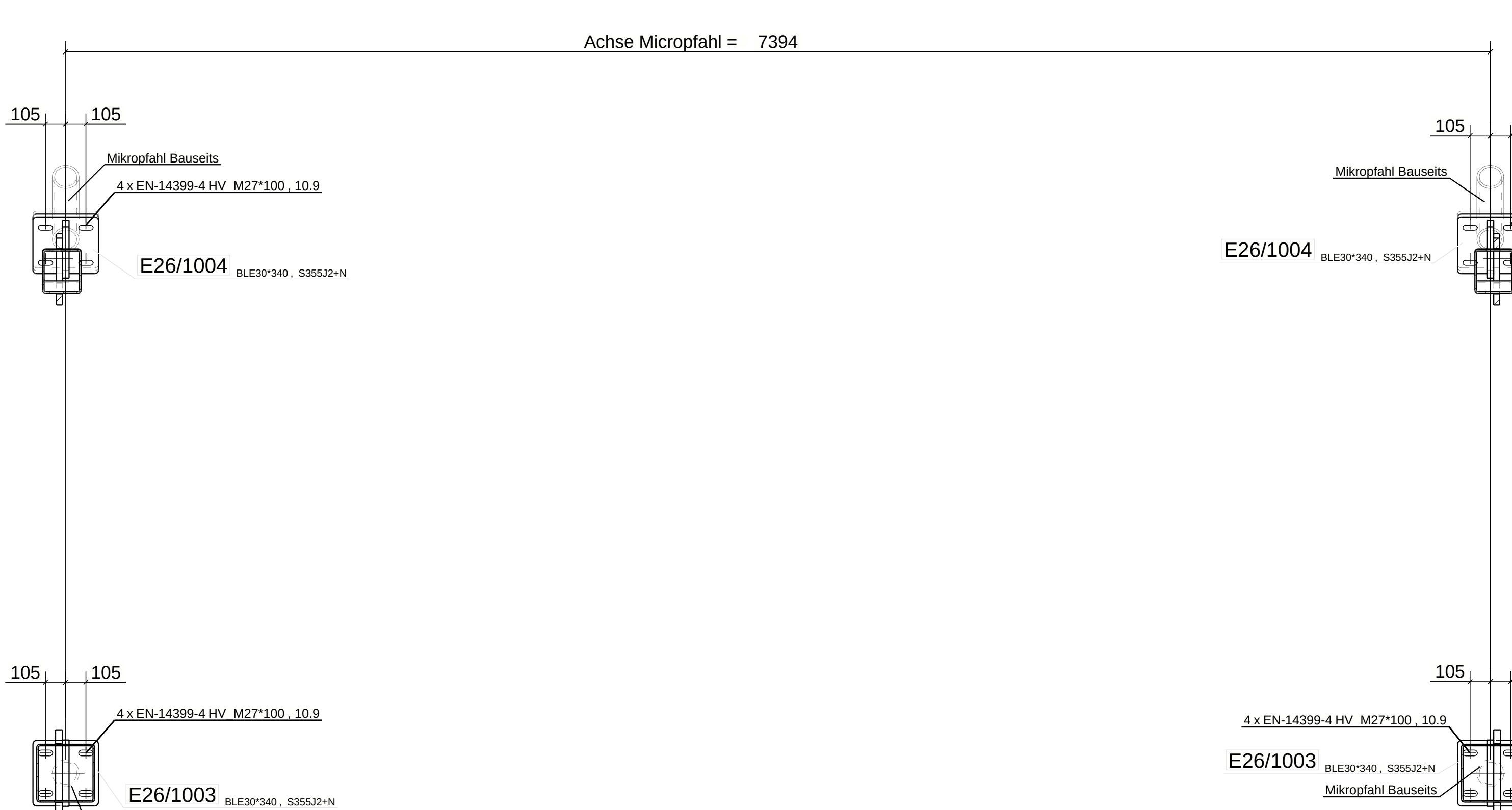
Grundriss: Primärkonstruktion Typ E - 2026
