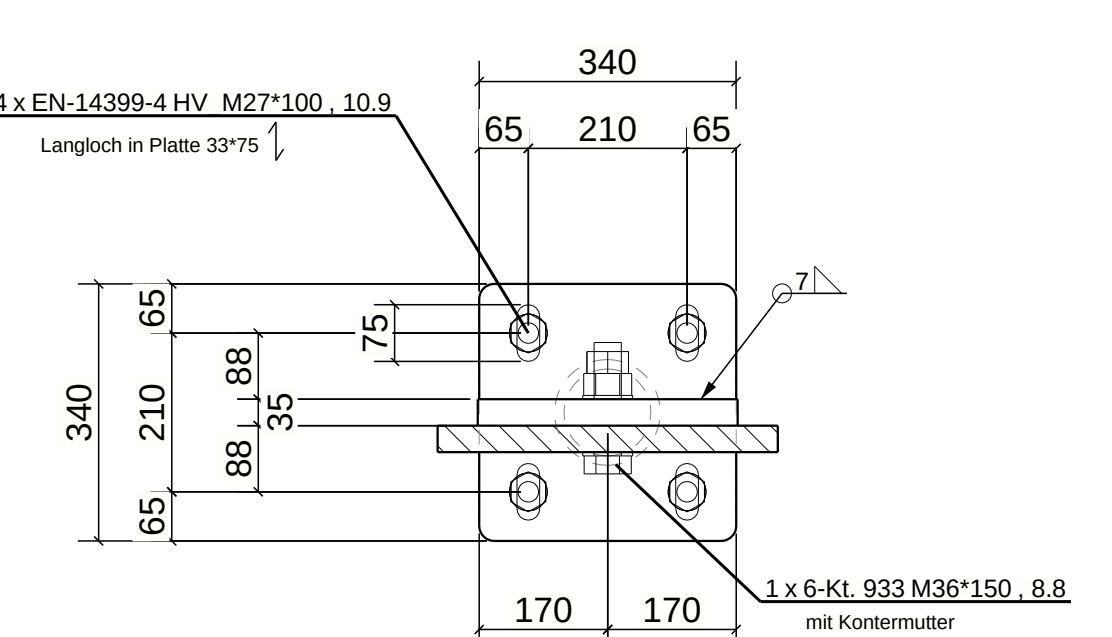
DETAIL 1, Schnitt C - C : talseitiger Stützenfuss (S1/S4)
