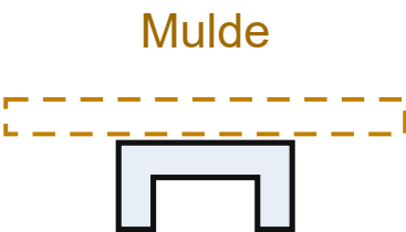
Pos 7 · U 100 längs unter die Mulde (2×)
