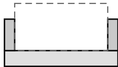
Pos 6 · Konsole Blech 10 mit Anschlag beidseits (4×)
